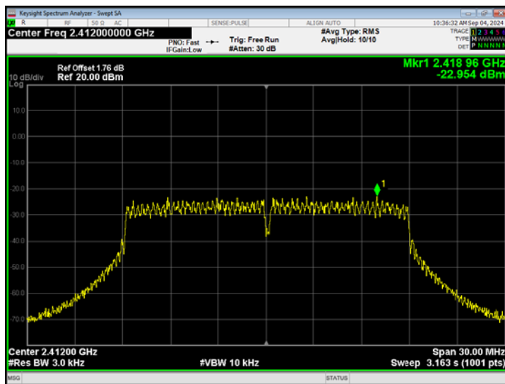
802.11n20 -CH01
