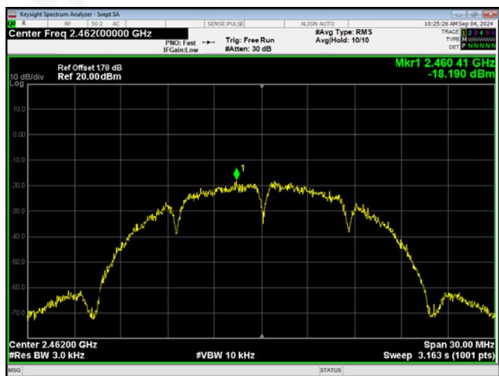
802.11b -CH11
