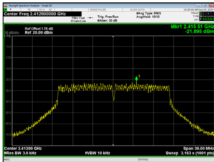
802.11g -CH01
