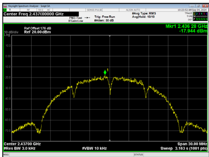
802.11b -CH06
