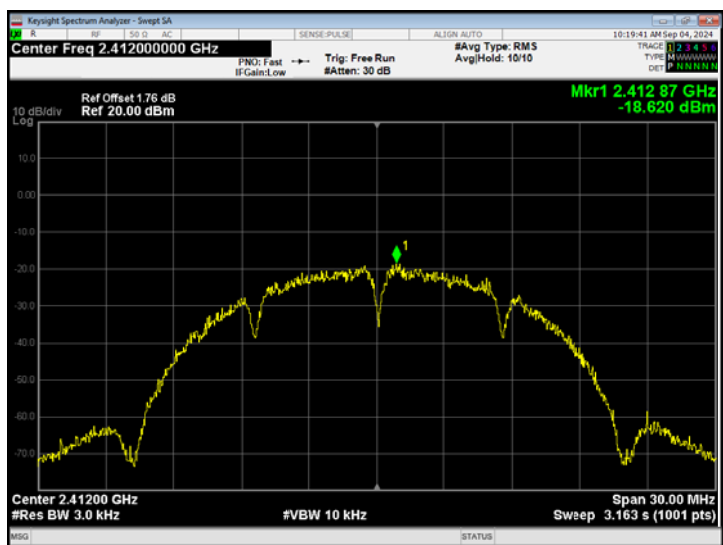
802.11b -CH01
