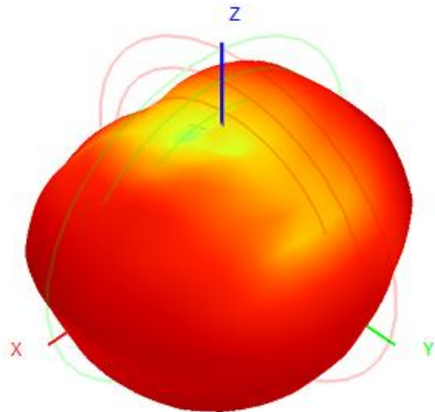
远场方向图
