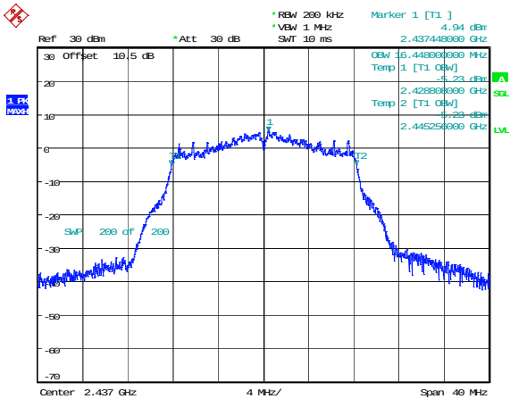
802.11g_2437MHz 16.448MHz
