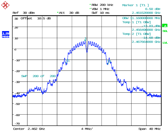
802.11b_2462MHz 11.168MHz
