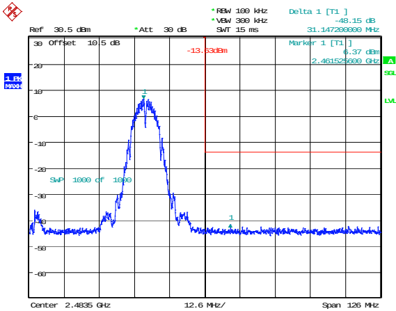
802.11b_2462MHz 48.15dB
