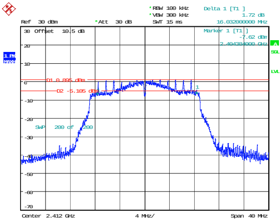
802.11n20_2412MHz 16.032MHz
