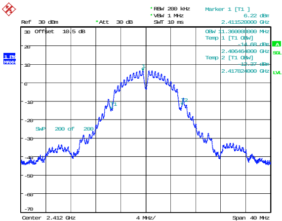
802.11b_2412MHz 11.360MHz
