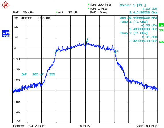
802.11g_2412MHz 16.448MHz
