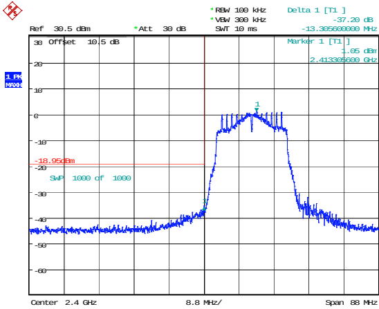
802.11n20_2412MHz 37.20dB
