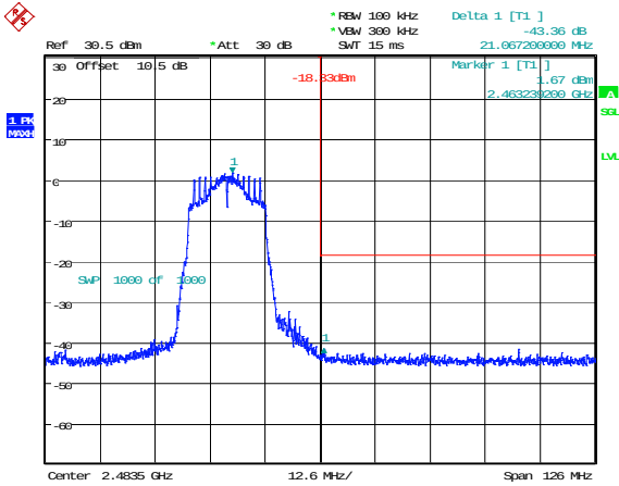
802.11n20_2462MHz 43.36dB
