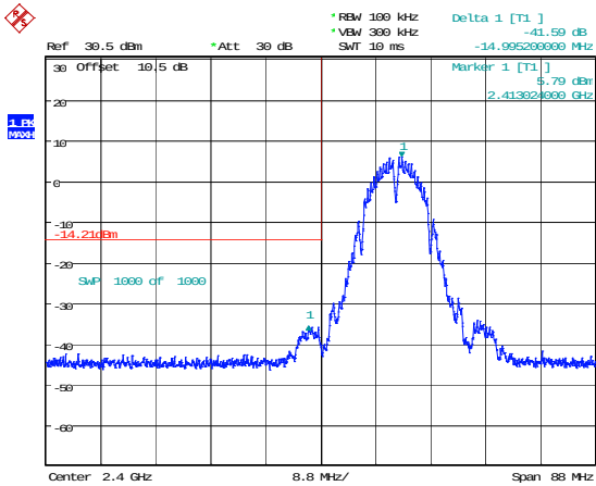
802.11b_2412MHz 41.59dB
