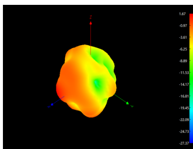
2450MHZ
