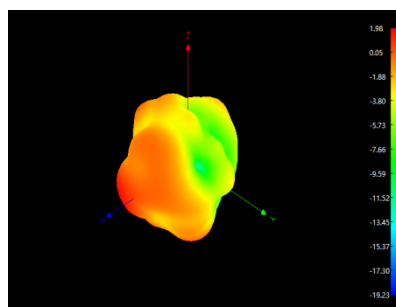
2500MHZ
