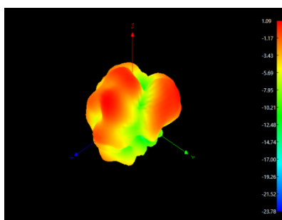
5500MHZ
