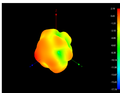
2400MHZ
