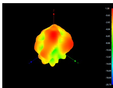
5850MHZ
