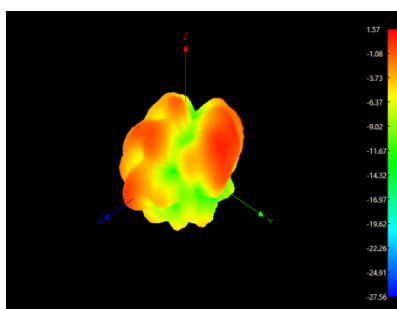
5150MHZ
