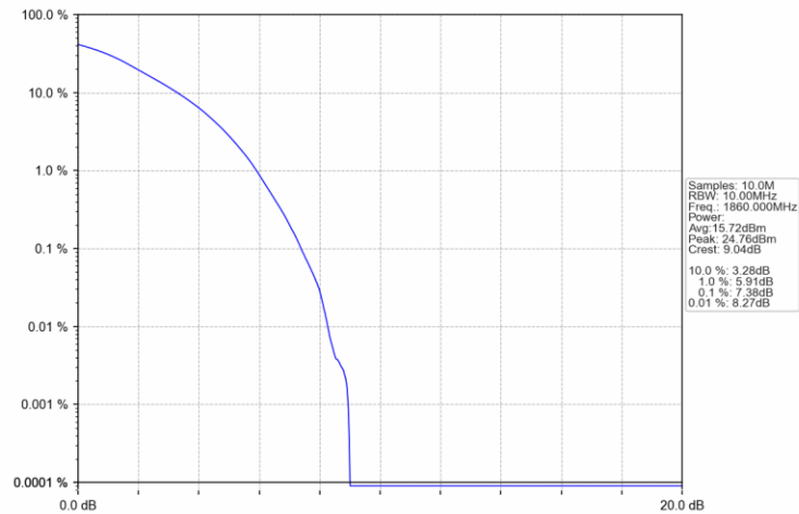
Band2_20MHz_16QAM_LCH_1860MHz_RB_27_0_NTNV
