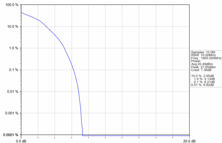
Band2_10MHz_16QAM_HCH_1905MHz_RB_27_23_NTNV
