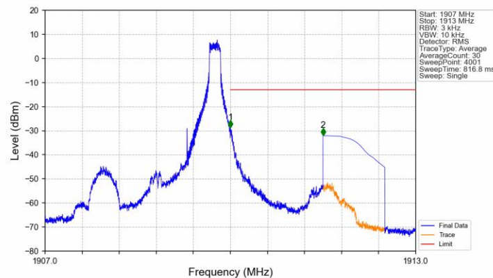
Band2_1.4MHz_QPSK_HCH_1909.3MHz_RB_1_5_NTNV
