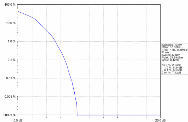
Band2_10MHz_16QAM_MCH_1880MHz_RB_27_0_NTNV
