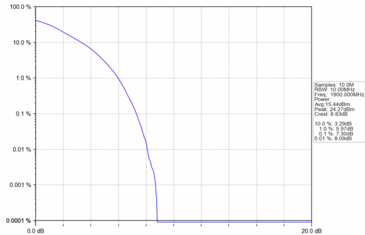
Band2_20MHz_16QAM_HCH_1900MHz_RB_27_73_NTNV
