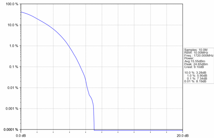
Band4_20MHz_16QAM_LCH_1720MHz_RB_27_0_NTNV
