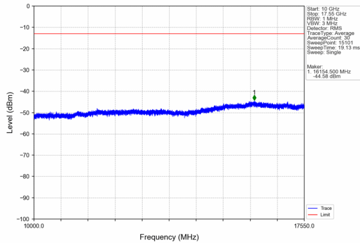
Band4_3MHz_QPSK_HCH_1753.5MHz_RB_1_14_NTNV
