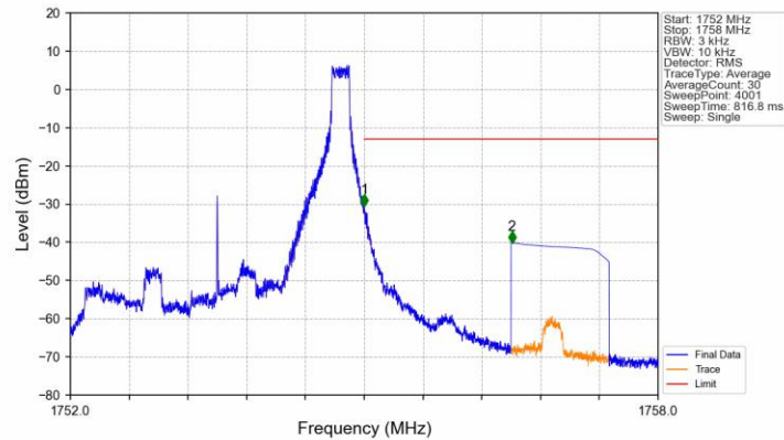
Band4_3MHz_QPSK_HCH_1753.5MHz_RB_1_14_NTNV
