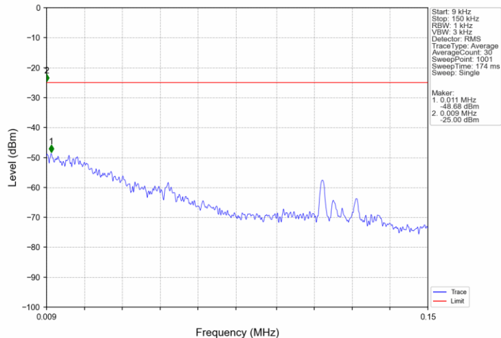
Band7_20MHz_QPSK_HCH_2560MHz_RB_1_0_NTNV
