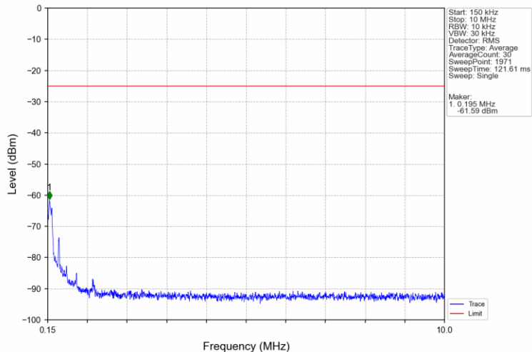
Band7_20MHz_QPSK_LCH_2510MHz_RB_1_0_NTNV
