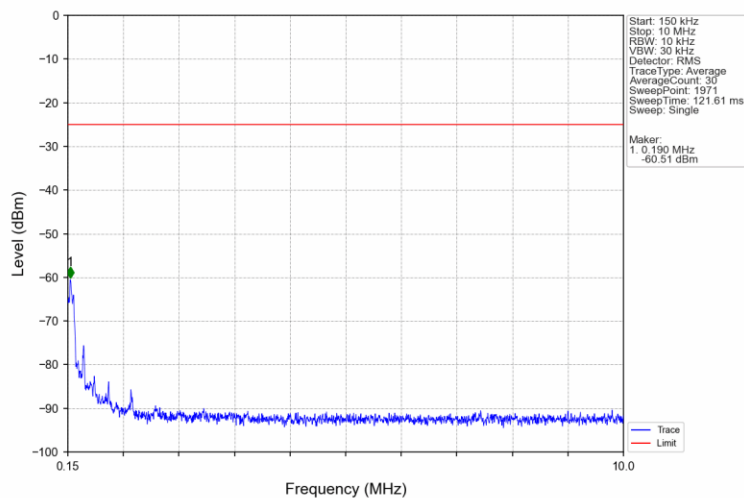
Band7_20MHz_QPSK_HCH_2560MHz_RB_1_0_NTNV
