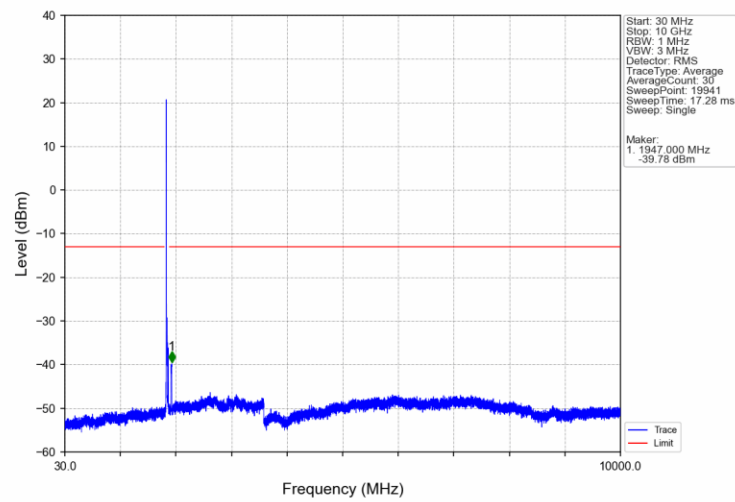
Band2_20MHz_16QAM_LCH_1860MHz_RB_1_0_NTNV
