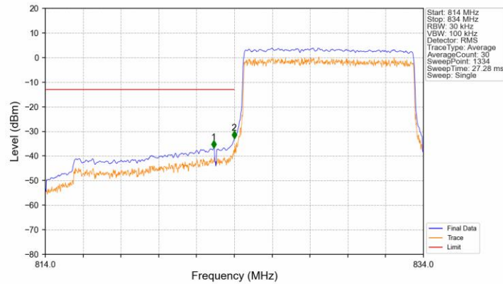
Band5_10MHz_QPSK_LCH_829MHz_RB_50_0_NTNV
