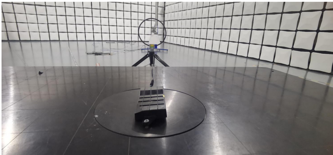
9KHz~30MHz
