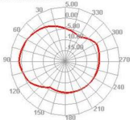
2500.000MHz H
