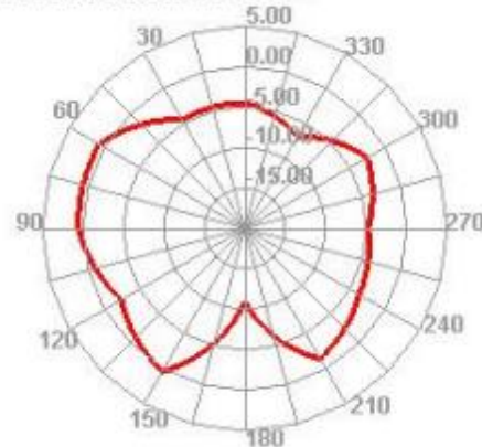
2450.000MHz E2
