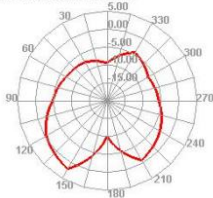
2500.000MHz E1
