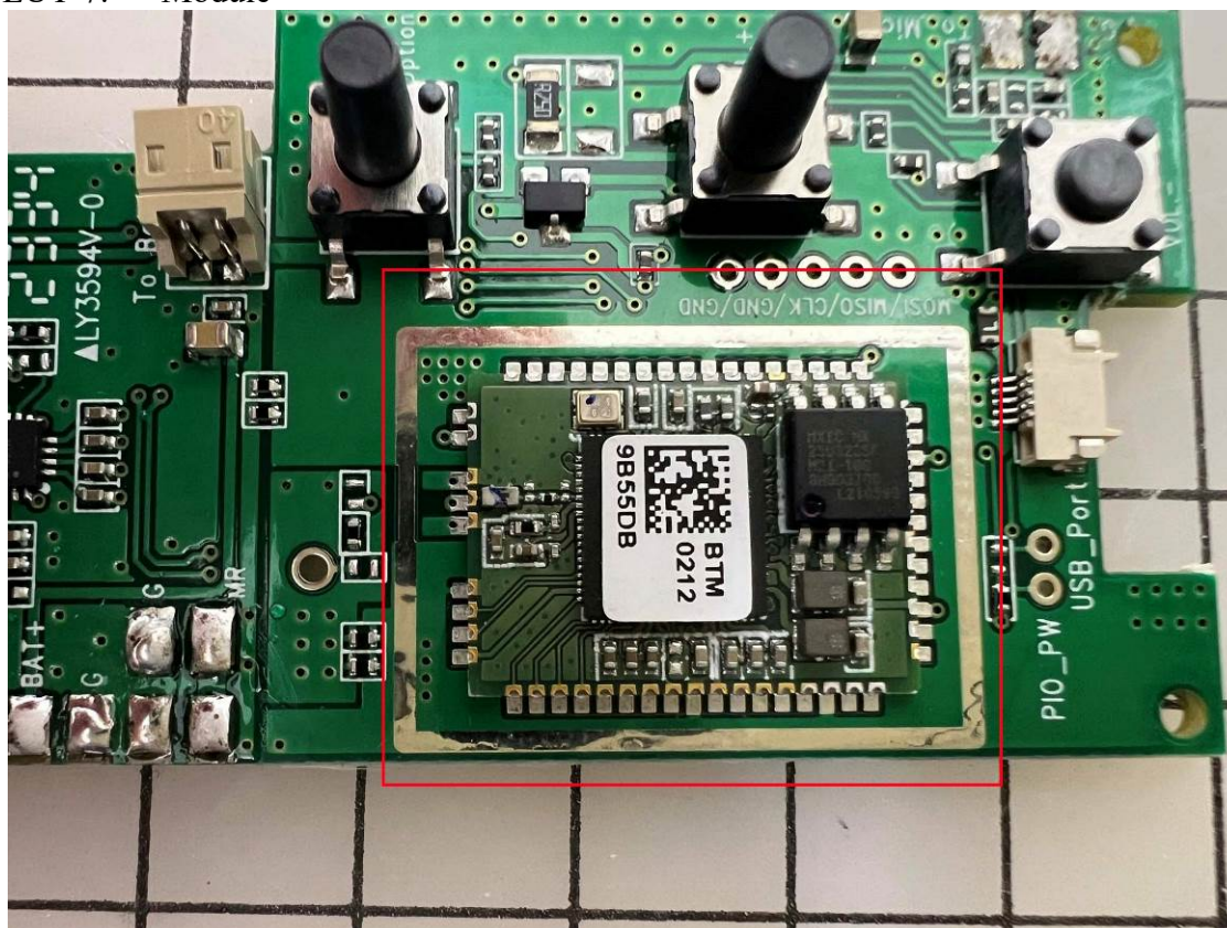
EUT-7. Module
