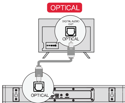
OPZIONE 1: OTTICO
