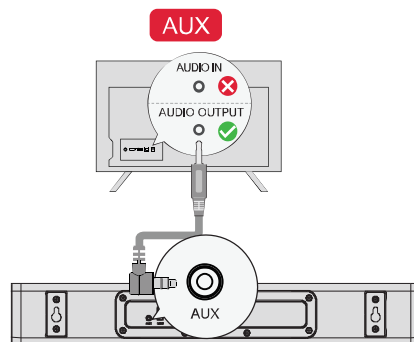
OPZIONE 2: AUX
