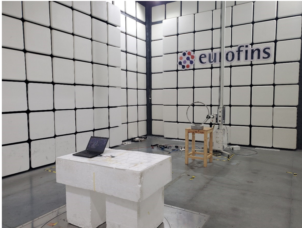
9kHz-30MHz
