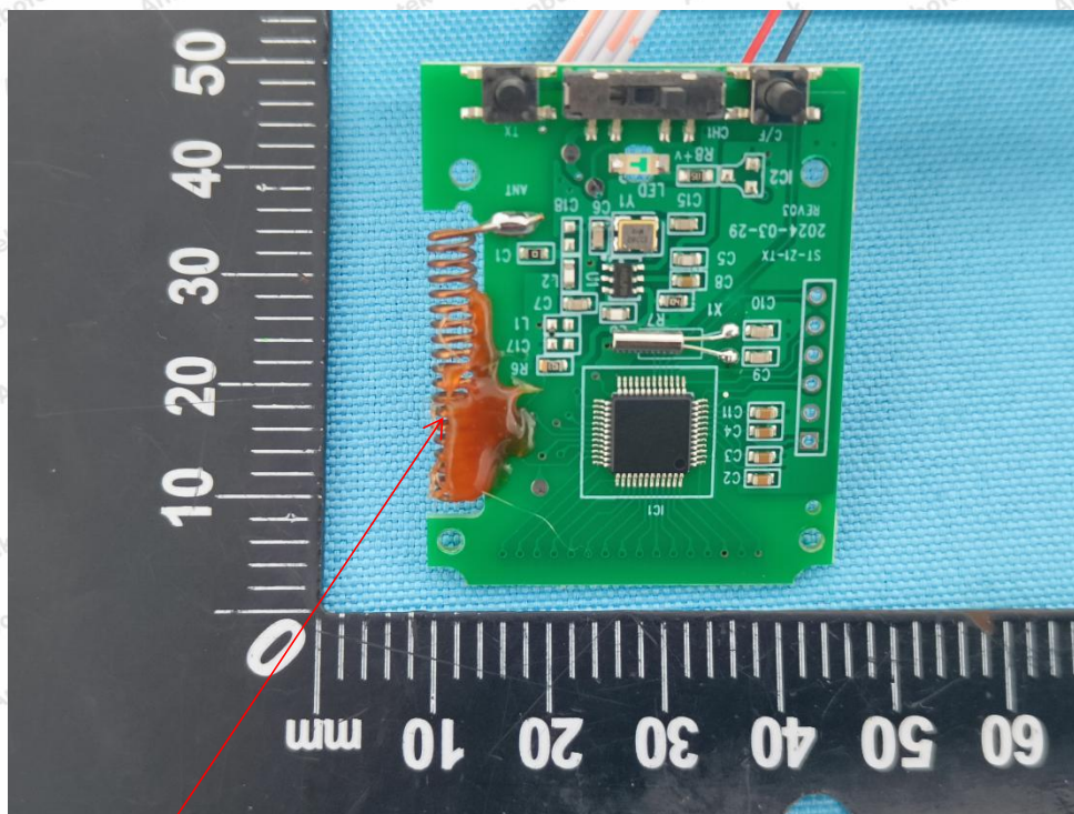
TX ANT
