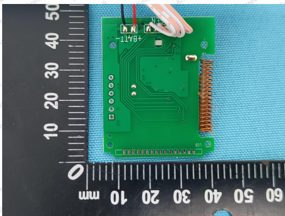
TX ANT
