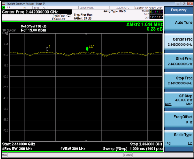
8DPSK
