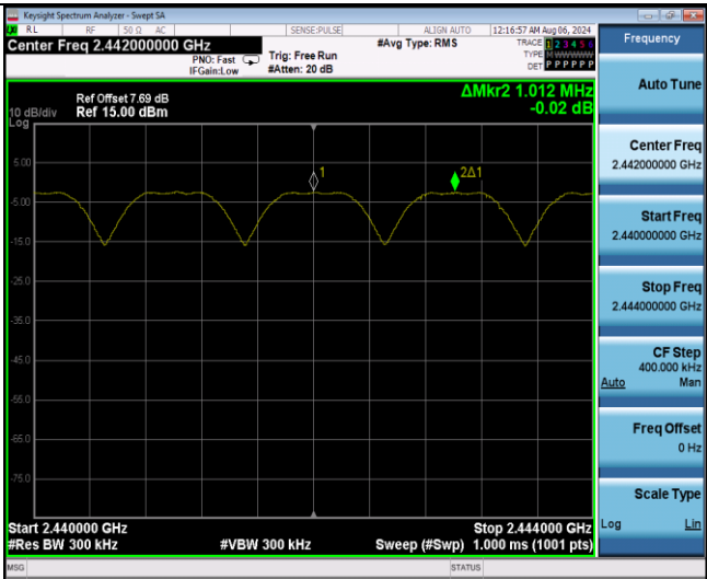
GFSK
