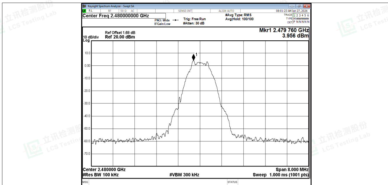
Band Edge NVNT BLE 1M 2480MHz Ant1 Ref
