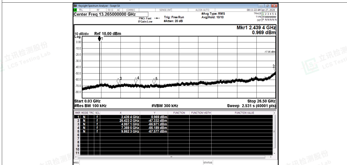
Tx. Spurious NVNT BLE 2M 2440MHz Ant1 Emission
