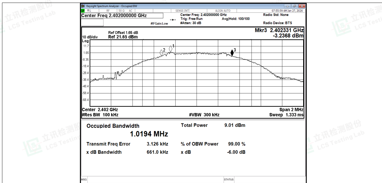
-6dB Bandwidth NVNT BLE 1M 2402MHz Ant1
