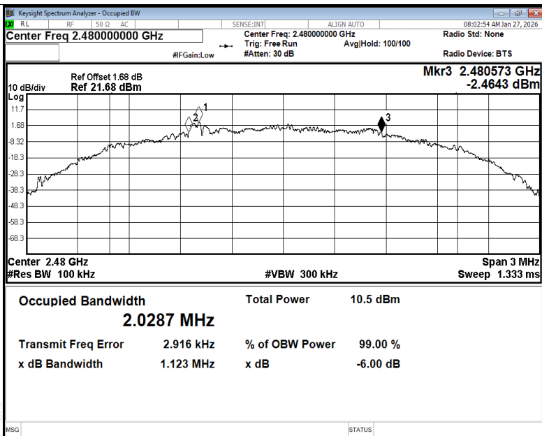
-6dB Bandwidth NVNT BLE 2M 2480MHz Ant1
