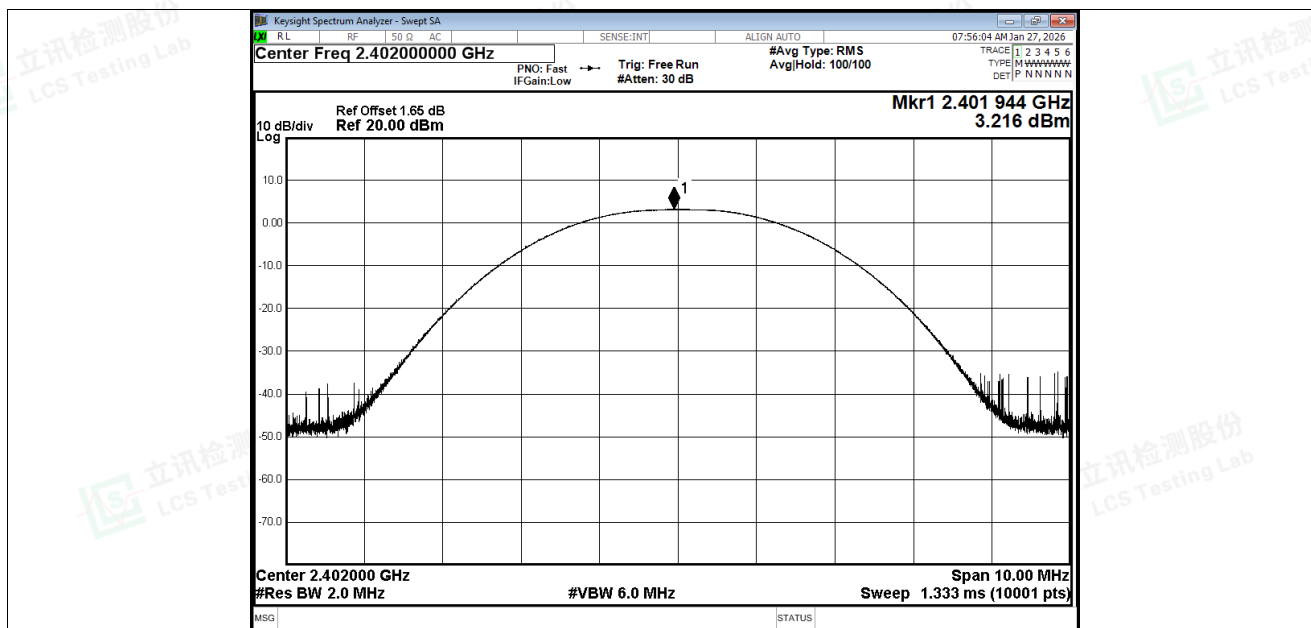
Peak Power NVNT BLE 1M 2402MHz Ant1
