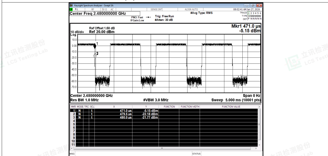
Duty Cycle NVNT BLE 2M 2480MHz Ant1
