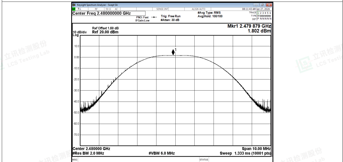
Peak Power NVNT BLE 2M 2480MHz Ant1
