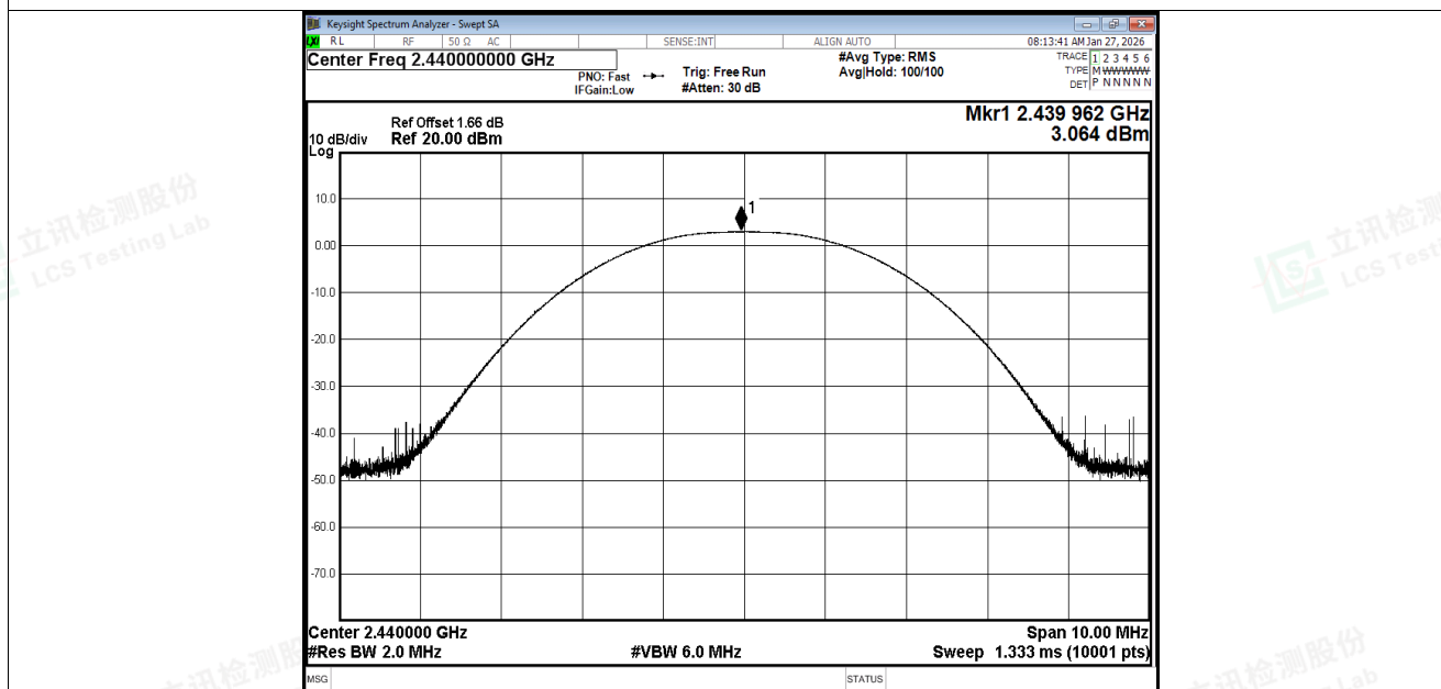
Peak Power NVNT BLE 1M 2440MHz Ant1
