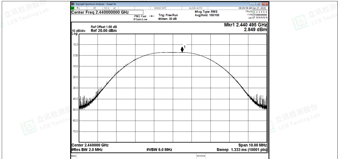
Peak Power NVNT BLE 2M 2440MHz Ant1
