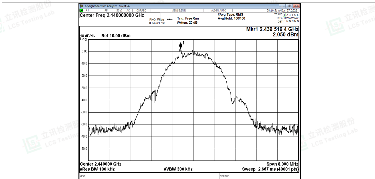
Tx. Spurious NVNT BLE 2M 2440MHz Ant1 Ref
