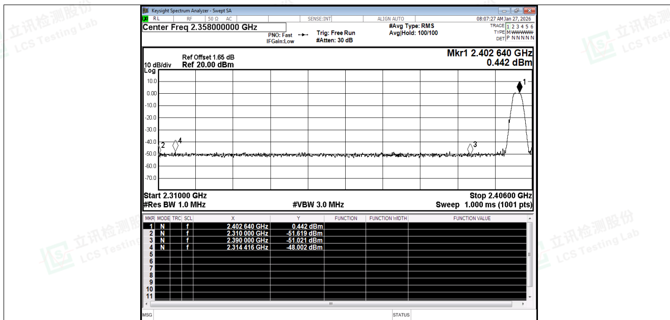
Restrict Band NVNT BLE 2M 2402MHz Ant1 Peak
