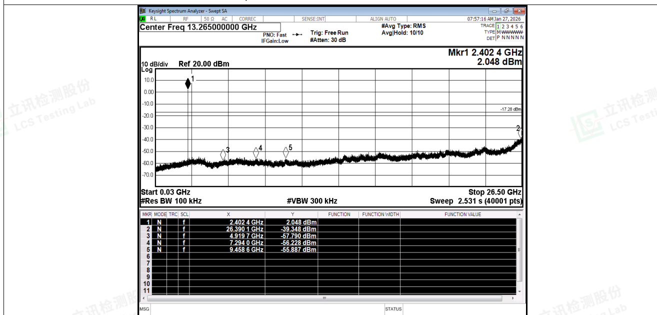
Tx. Spurious NVNT BLE 1M 2402MHz Ant1 Emission
