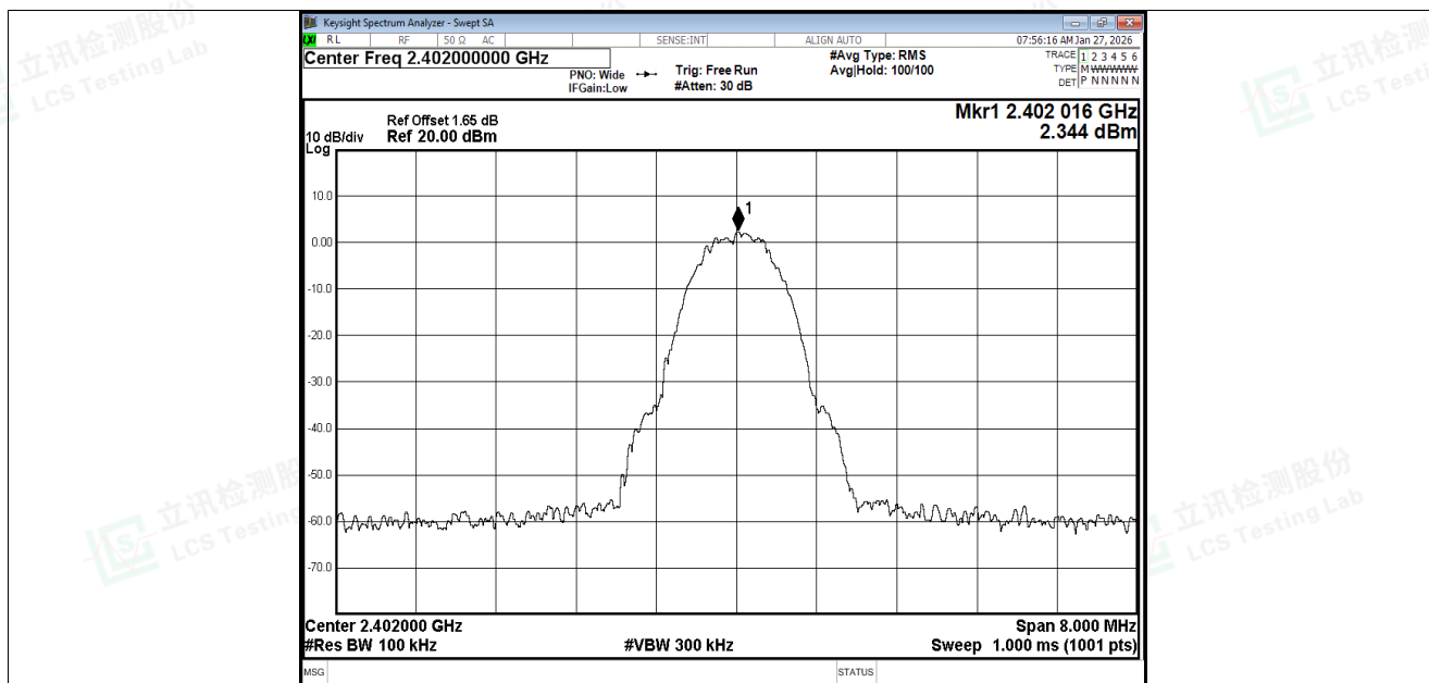
Band Edge NVNT BLE 1M 2402MHz Ant1 Ref
