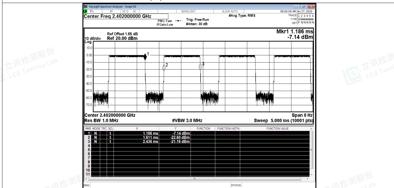
Duty Cycle NVNT BLE 2M 2402MHz Ant1
