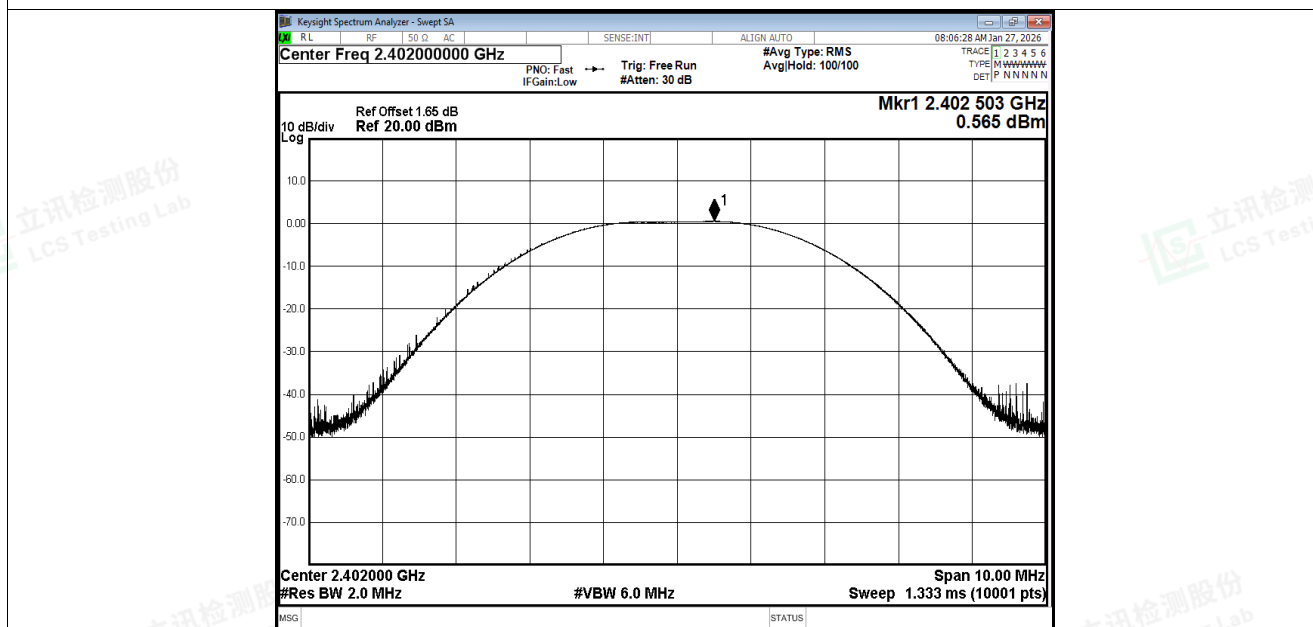
Peak Power NVNT BLE 2M 2402MHz Ant1
