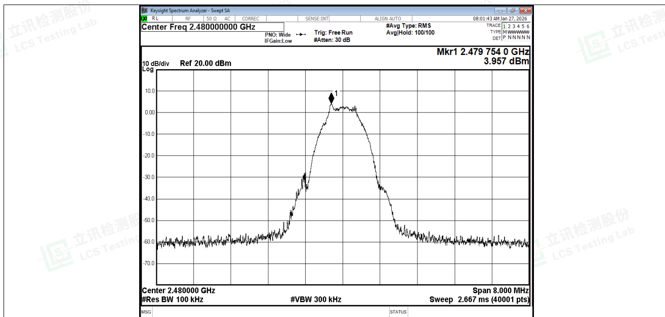
Tx. Spurious NVNT BLE 1M 2480MHz Ant1 Ref
