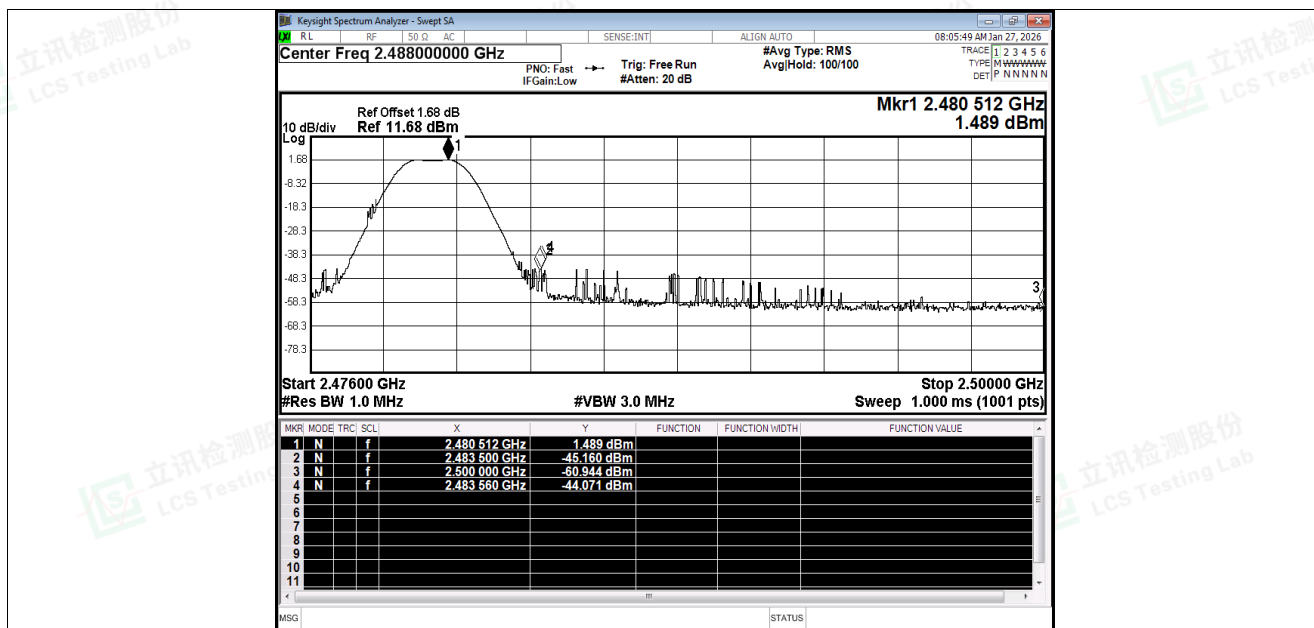
Restrict Band NVNT BLE 2M 2480MHz Ant1 Peak
