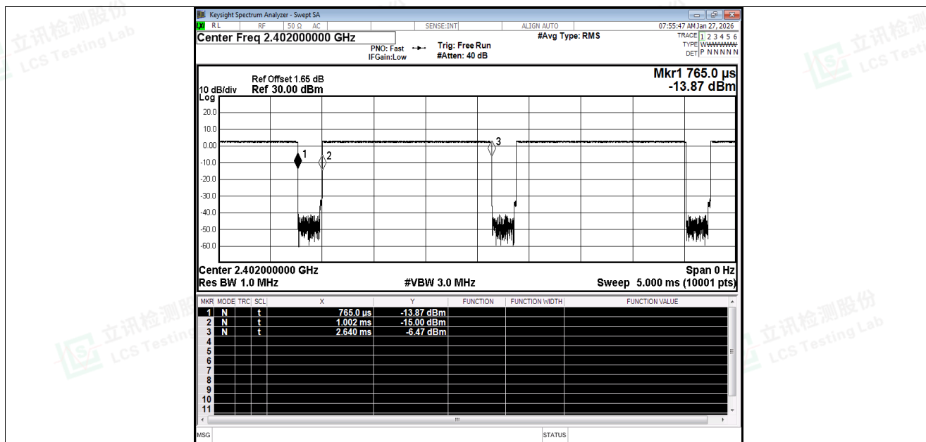
Duty Cycle NVNT BLE 1M 2402MHz Ant1
