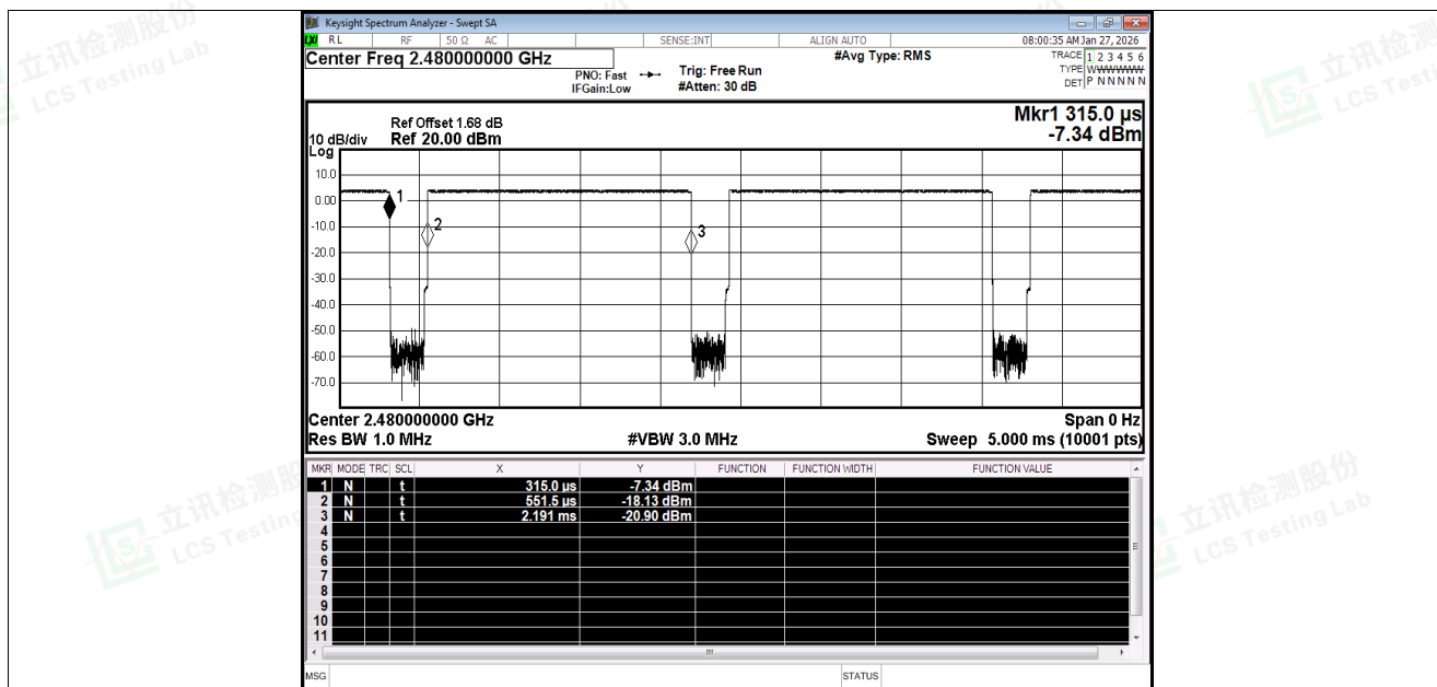
Duty Cycle NVNT BLE 1M 2480MHz Ant1
