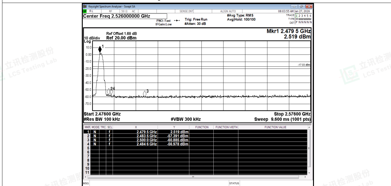
Band Edge NVNT BLE 2M 2480MHz Ant1 Emission
