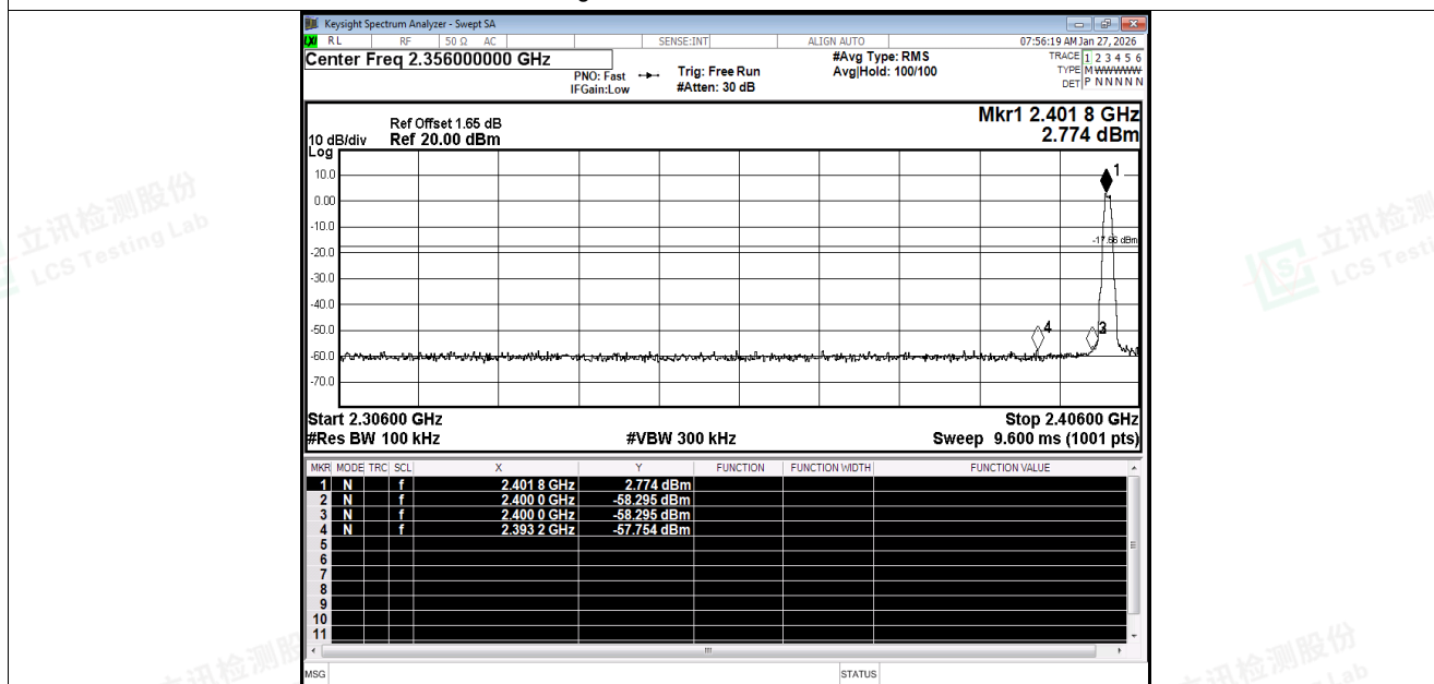
Band Edge NVNT BLE 1M 2402MHz Ant1 Emission
