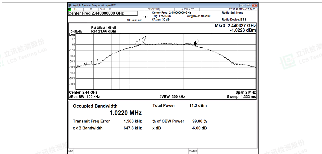
-6dB Bandwidth NVNT BLE 1M 2440MHz Ant1
