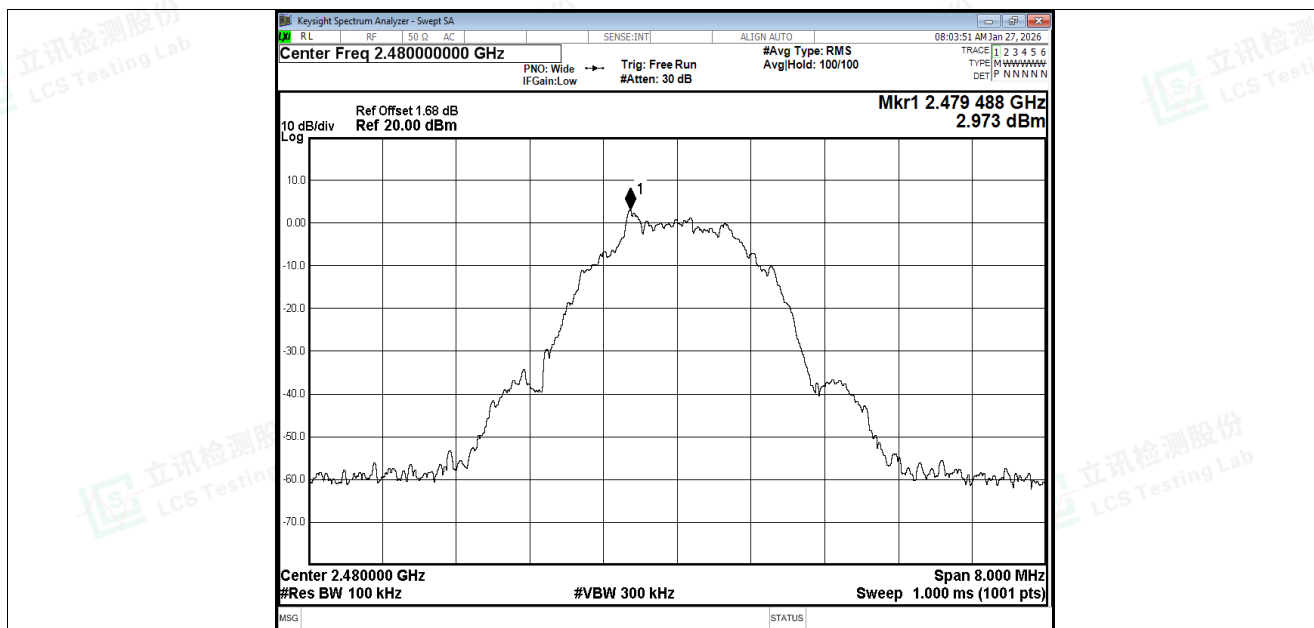
Band Edge NVNT BLE 2M 2480MHz Ant1 Ref
