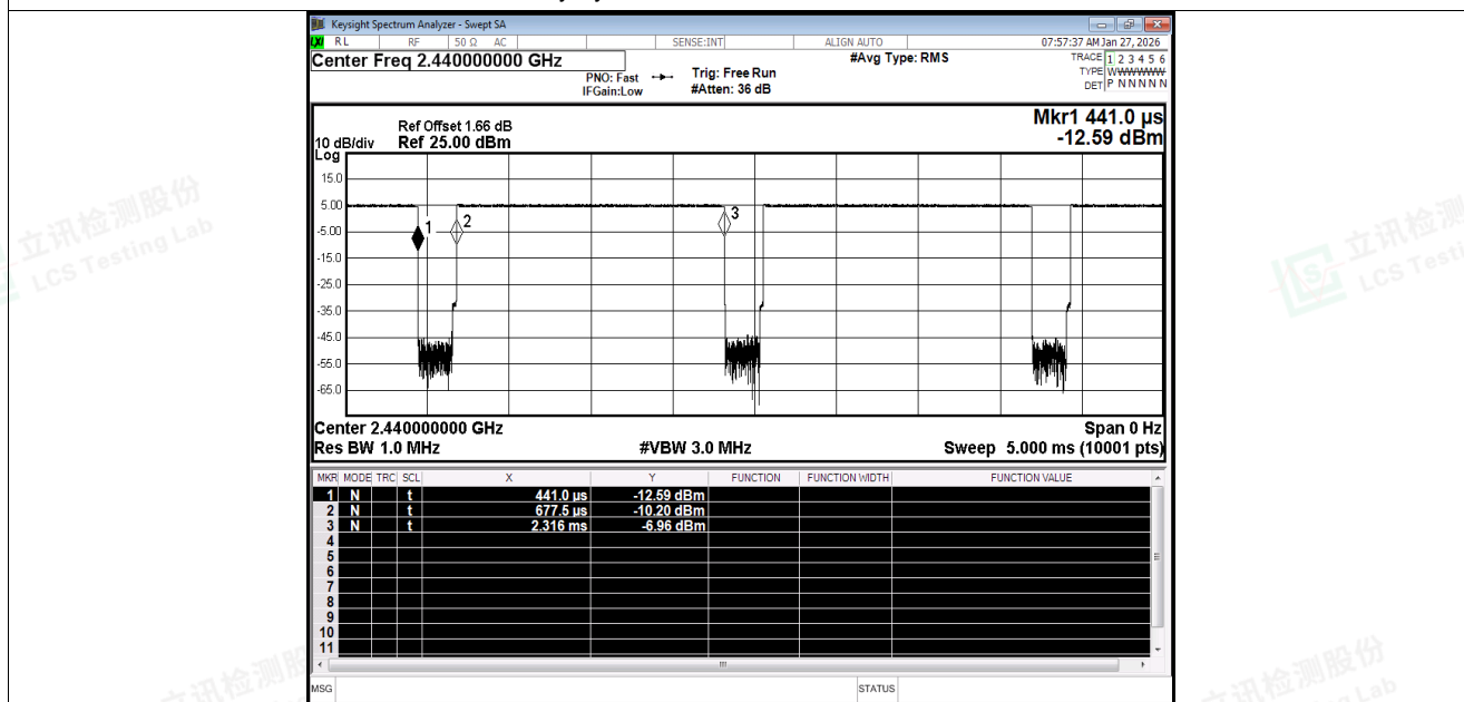
Duty Cycle NVNT BLE 1M 2440MHz Ant1
