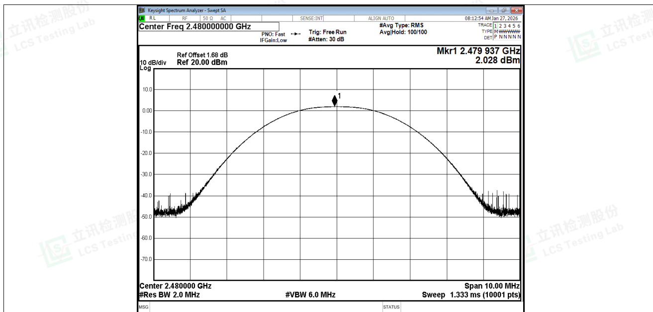
Peak Power NVNT BLE 1M 2480MHz Ant1
