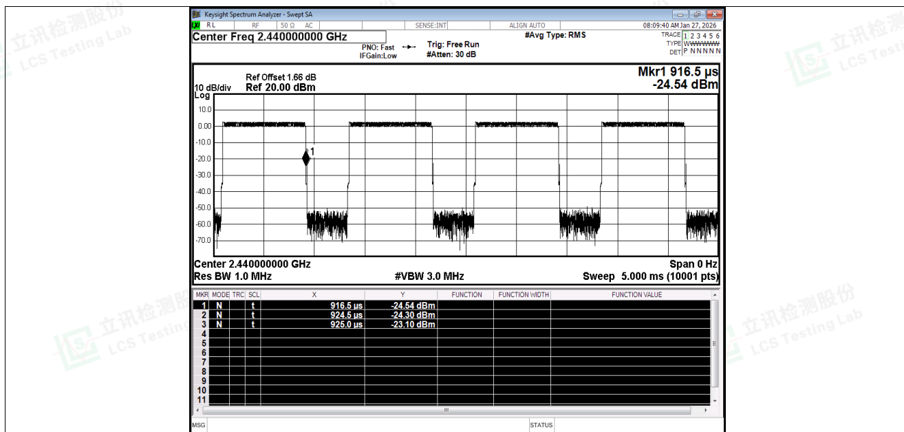
Duty Cycle NVNT BLE 2M 2440MHz Ant1
