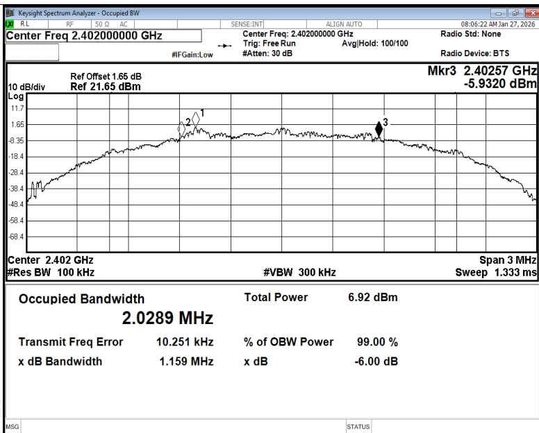
-6dB Bandwidth NVNT BLE 2M 2402MHz Ant1
