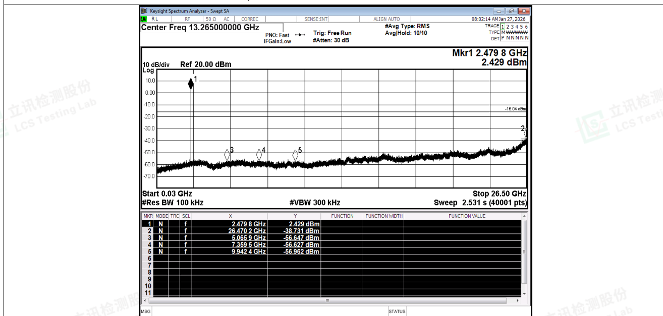
Tx. Spurious NVNT BLE 1M 2480MHz Ant1 Emission
