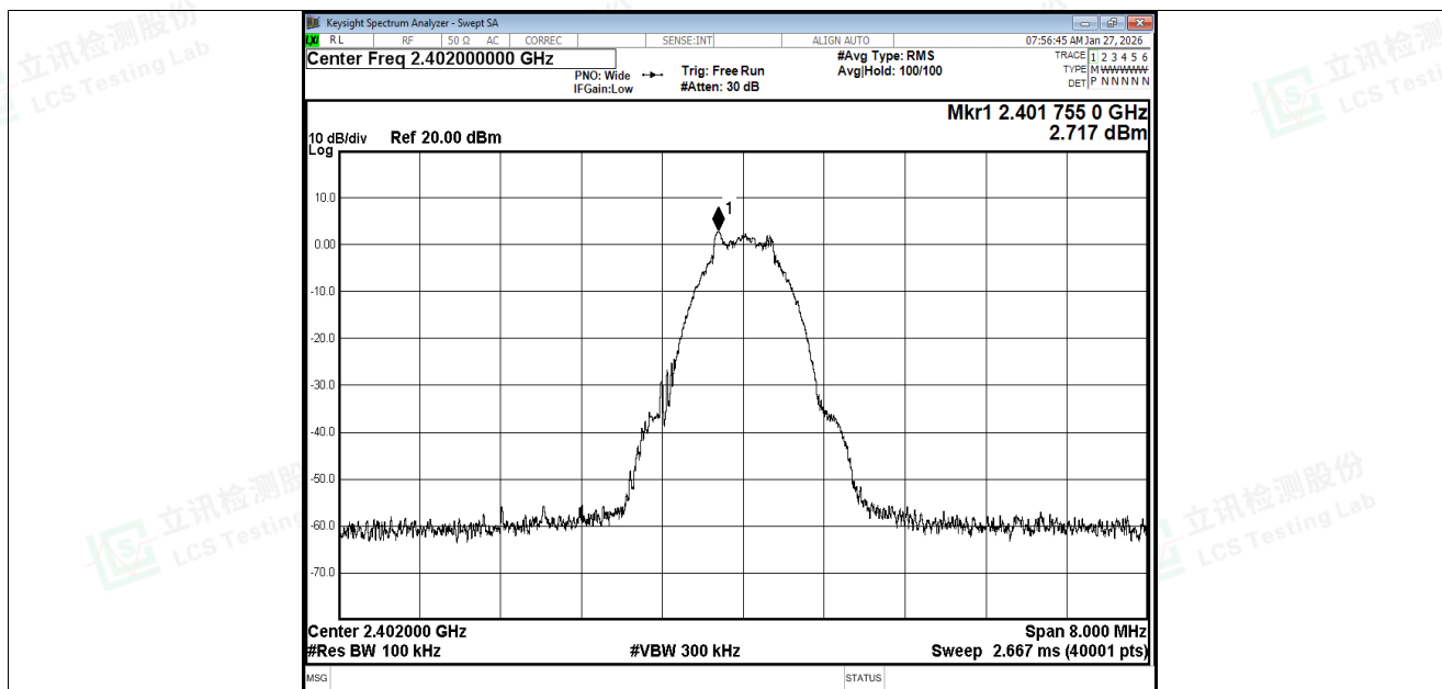
Tx. Spurious NVNT BLE 1M 2402MHz Ant1 Ref
