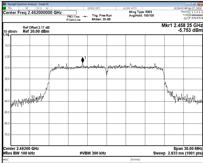
Band Edge NVNT n20 2462MHz Ant1 Ref
