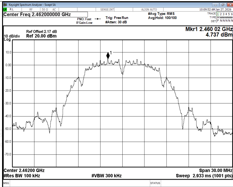
Band Edge NVNT b 2462MHz Ant1 Ref
