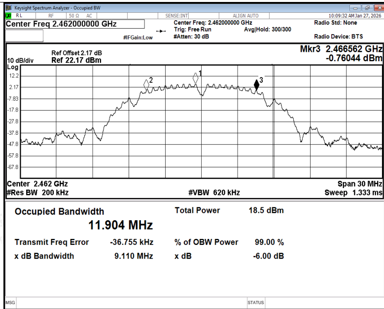
-6dB Bandwidth NVNT b 2462MHz Ant1
