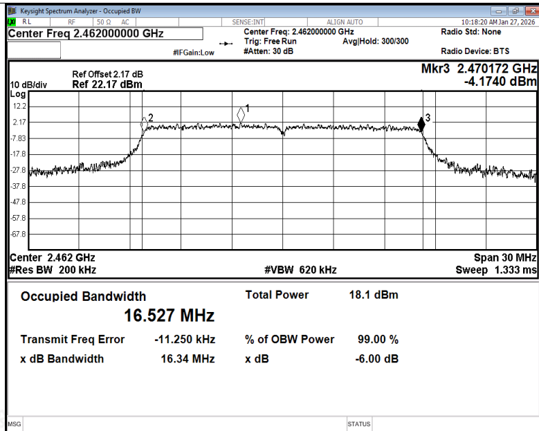
-6dB Bandwidth NVNT g 2462MHz Ant1
