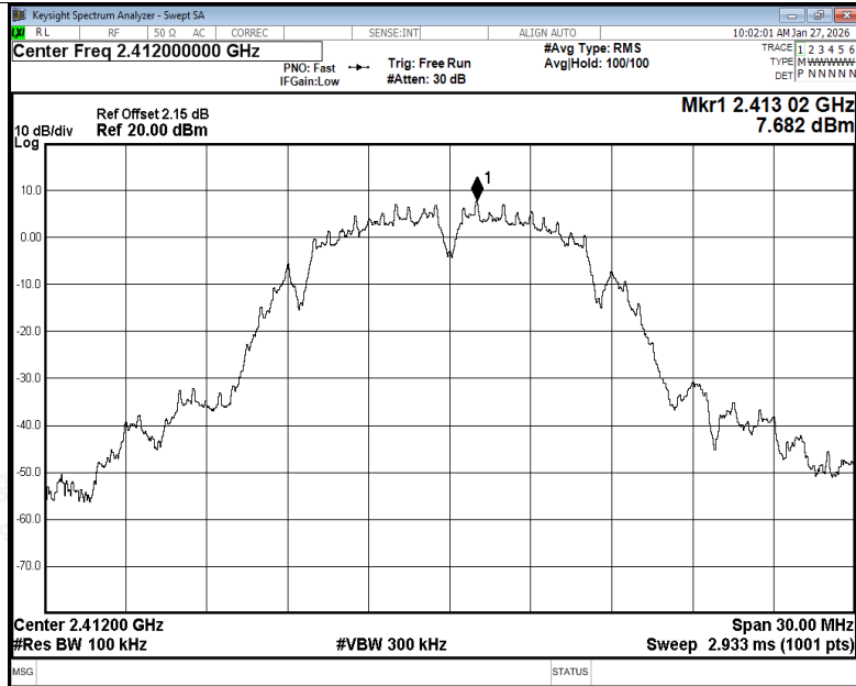
Band Edge NVNT b 2412MHz Ant1 Ref
