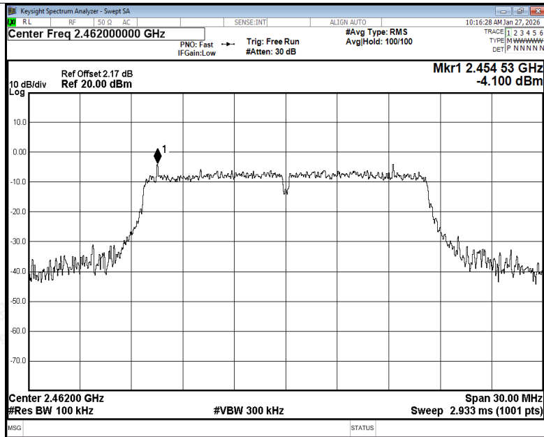
Band Edge NVNT g 2462MHz Ant1 Ref
