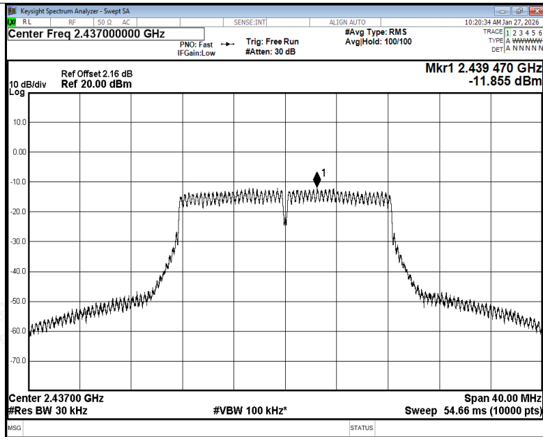
PSD NVNT g 2437MHz Ant1
