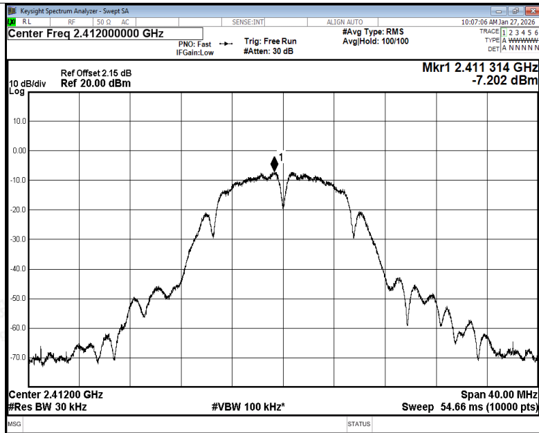
PSD NVNT b 2412MHz Ant1
