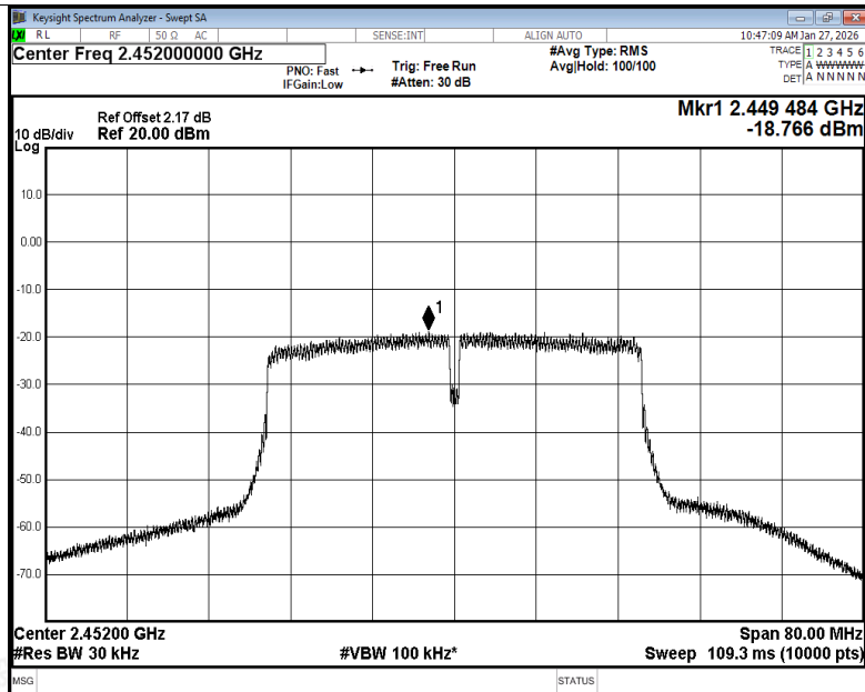
PSD NVNT n40 2452MHz Ant1
