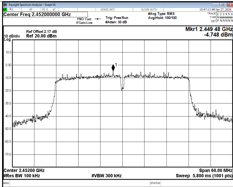
Band Edge NVNT n40 2452MHz Ant1 Ref
