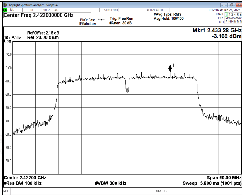
Band Edge NVNT n40 2422MHz Ant1 Ref
