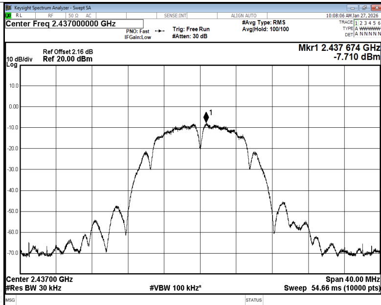
PSD NVNT b 2437MHz Ant1
