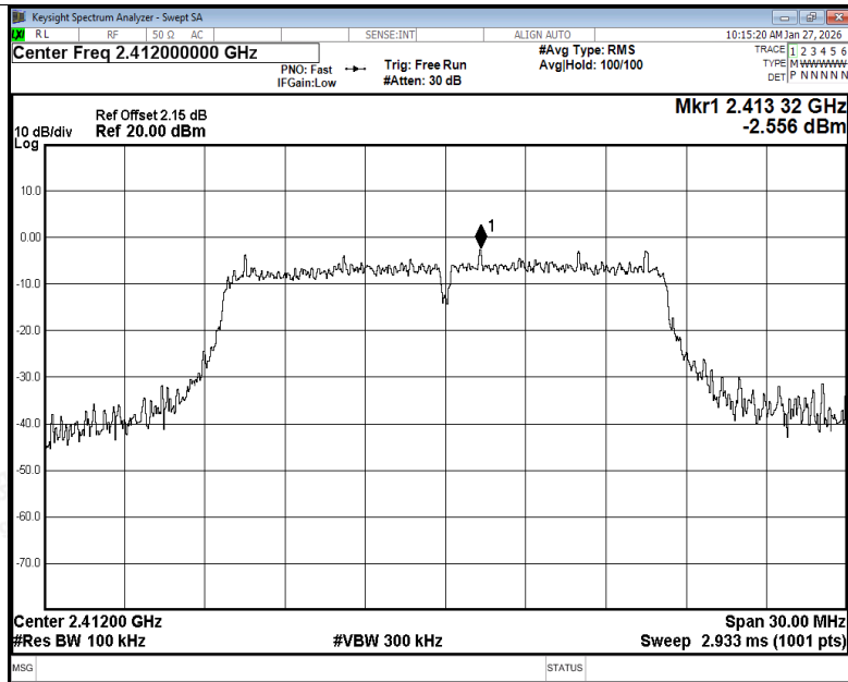
Band Edge NVNT g 2412MHz Ant1 Ref
