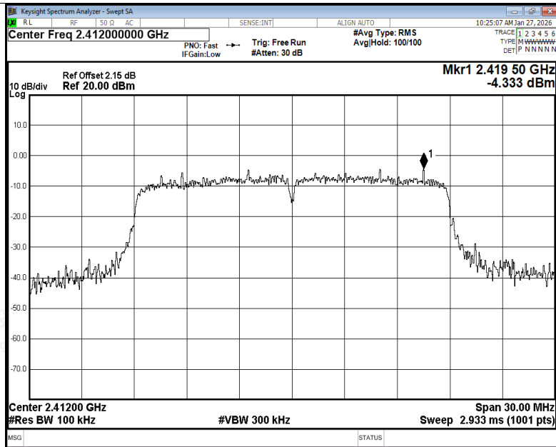
Band Edge NVNT n20 2412MHz Ant1 Ref
