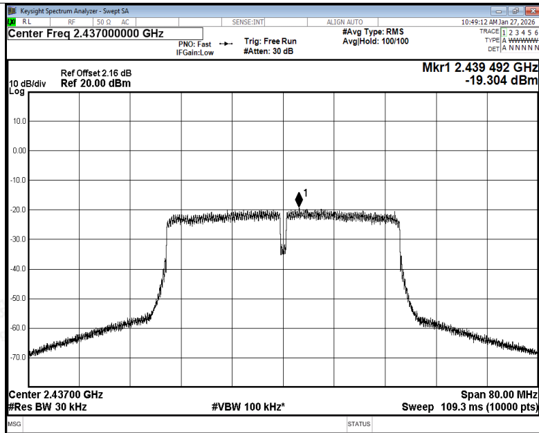
PSD NVNT n40 2437MHz Ant1
