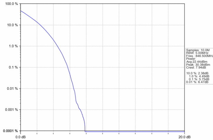
Band26b 5MHz QPSK HCH 846.5MHz RB 25 0 NTNV
