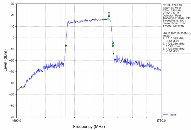
Band4 20MHz 16QAM LCH 1720MHz RB 100 0 NTV
