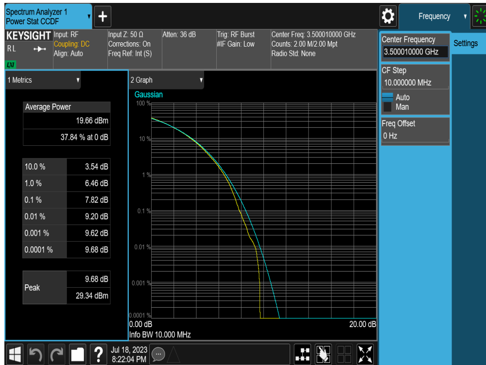
Plot 7-51. PAR Plot (NR Band n78 - 10MHz CP-OFDM 256-QAM-- Full RB)
