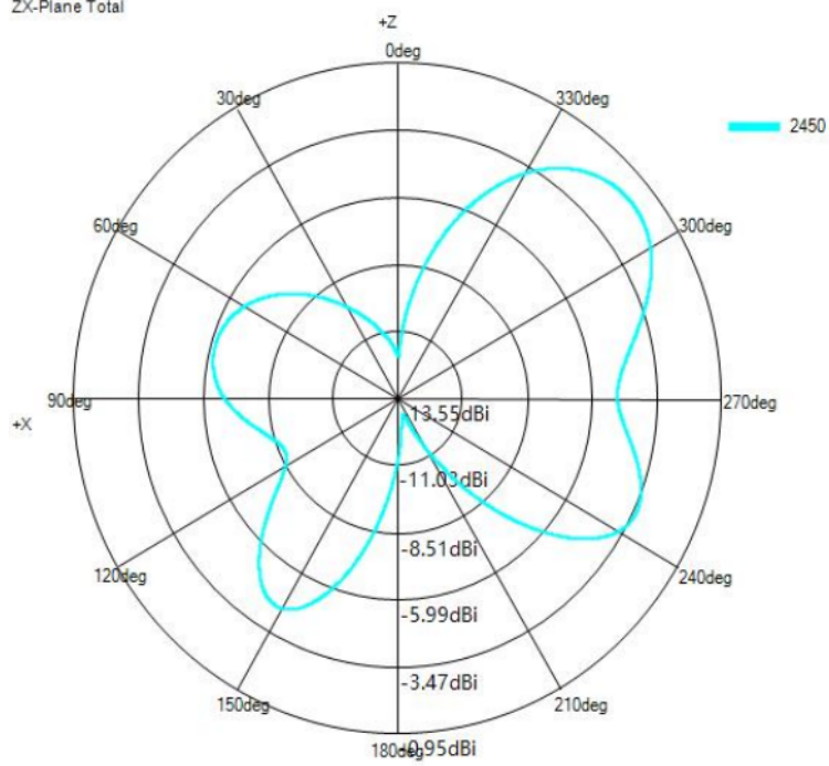
ZX-Plane Total
