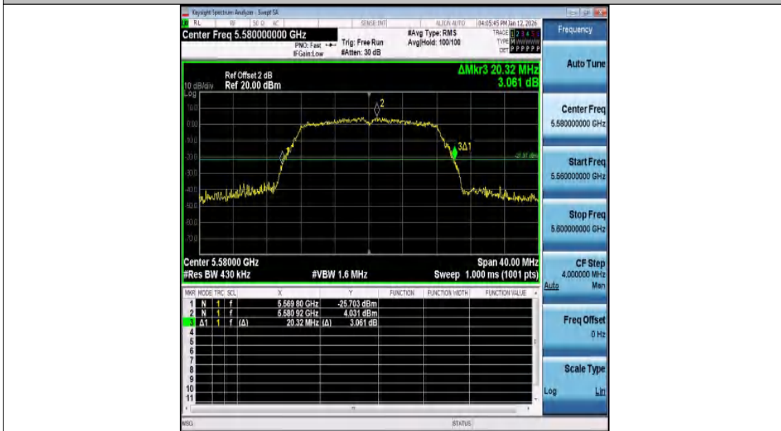
11A-Ant1-5580
