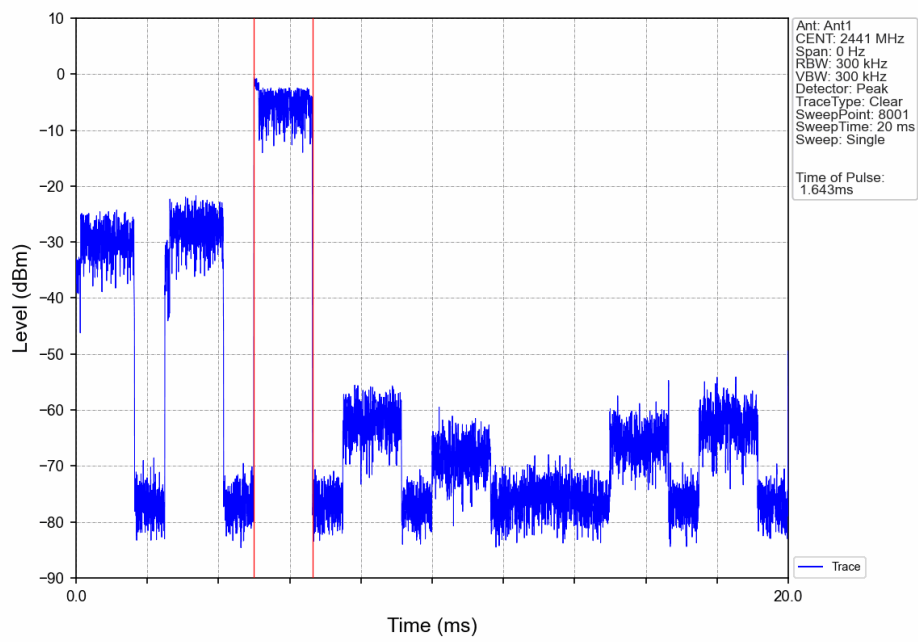
Pi/4DQPSK_2DH3_HOPP_Ant1_NTNV
