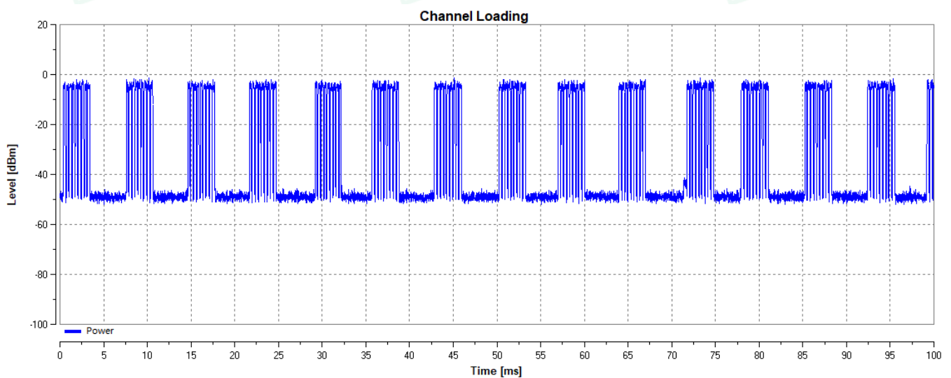
802.11ac VHT40
