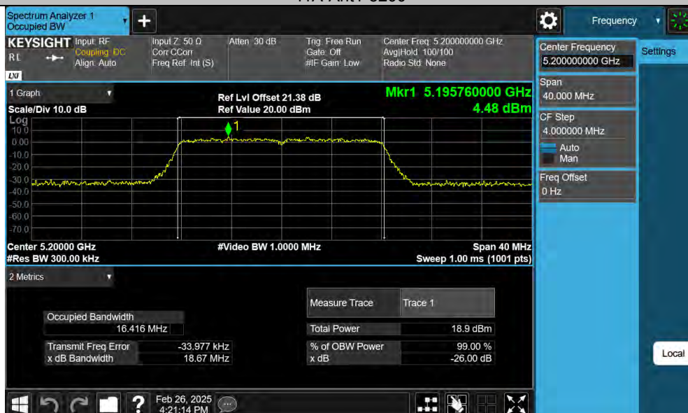
11A-Ant1-5200
