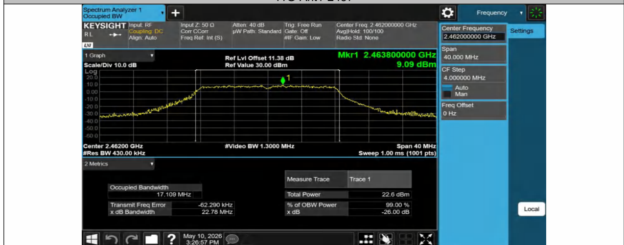
11G-Ant1-2462
