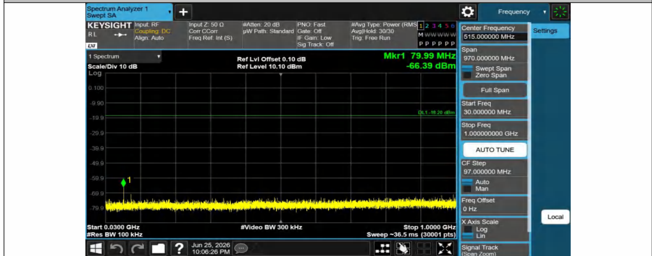
11G-Ant1-2462-30~1000-PASS
