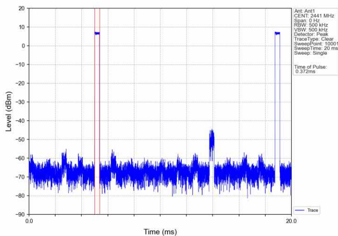
GFSK_DH1_HOPP_Ant1_NTNV
