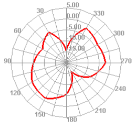
5150.000MHz E1
