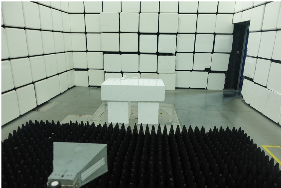
1GHz-18GHz
