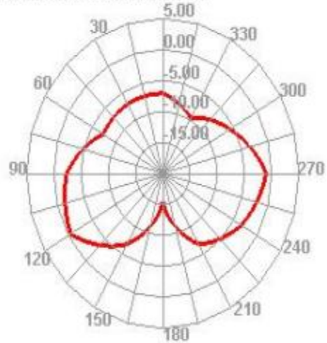
2420.000MHz E2
