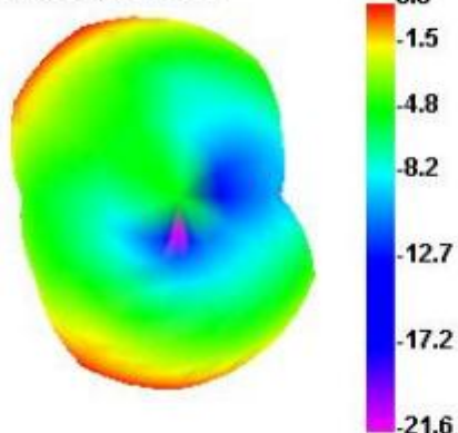
2480.000MHz
