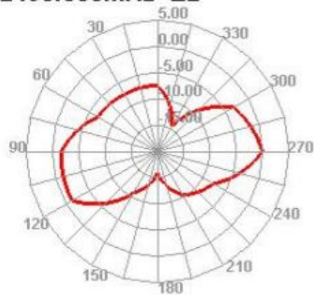
2490.000MHz E2
