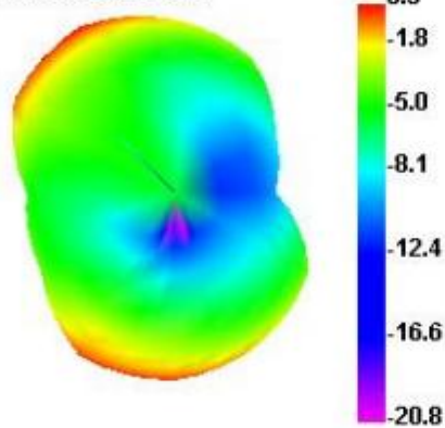
2490.000MHz
