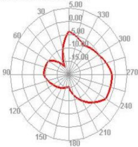
2420.000MHz E1
