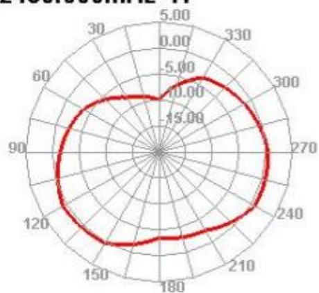
2490.000MHz H
