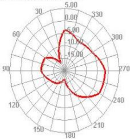
2410.000MHz E1
