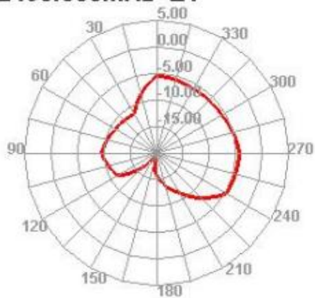
2490.000MHz E1
