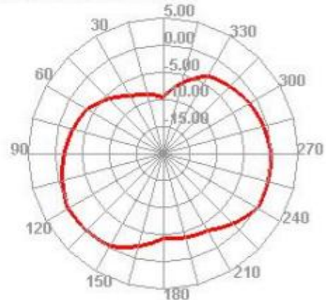
2490.000MHz H
