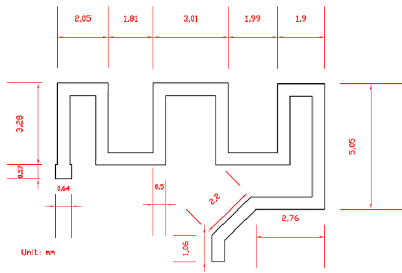
图 1 尺寸图 Figure 1 Size diagram
