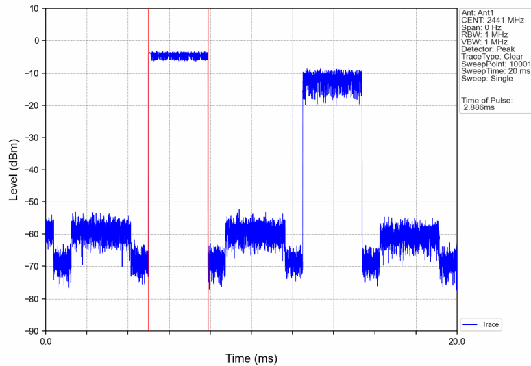
Pi/4DQPSK_2DH5_HOPP_Ant1_NTNV
