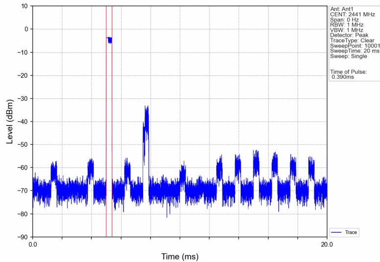
Pi/4DQPSK_2DH1_HOPP_Ant1_NTNV
