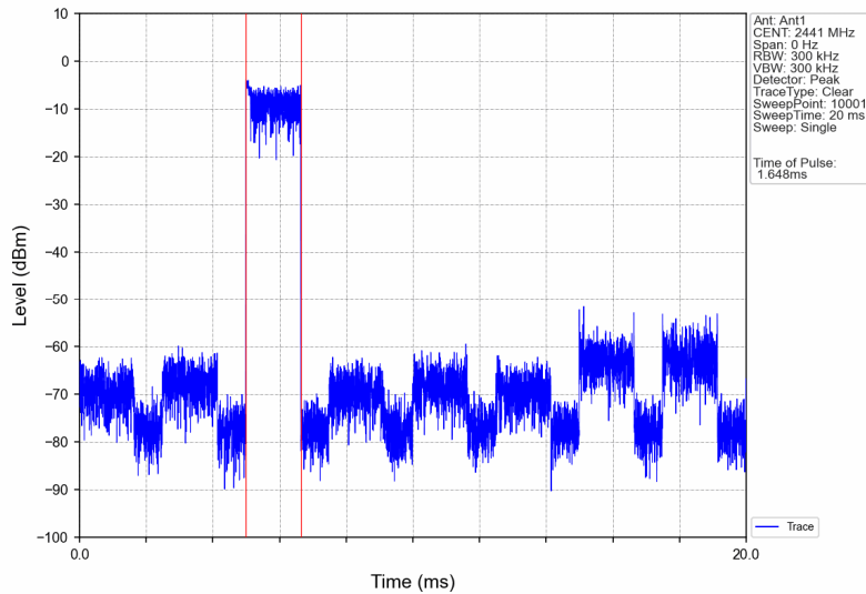
8DPSK_3DH3_HOPP_Ant1_NTNV
