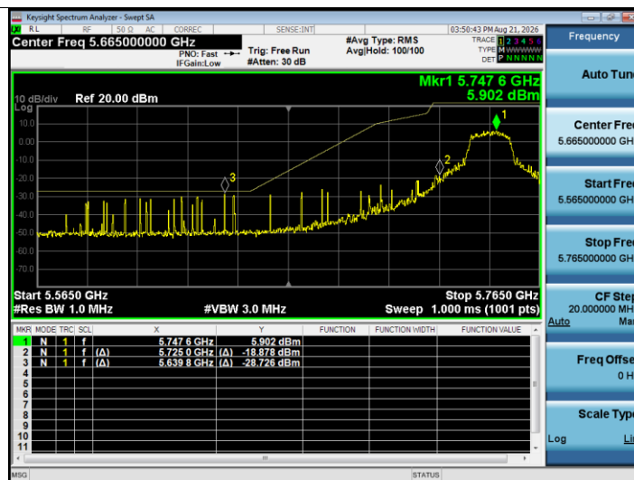
Band Edge NVNT 5745MHz Low Ant1
