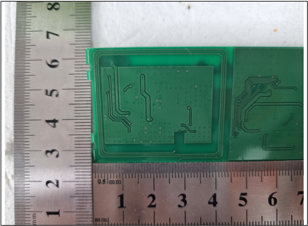
NFC Antenna
