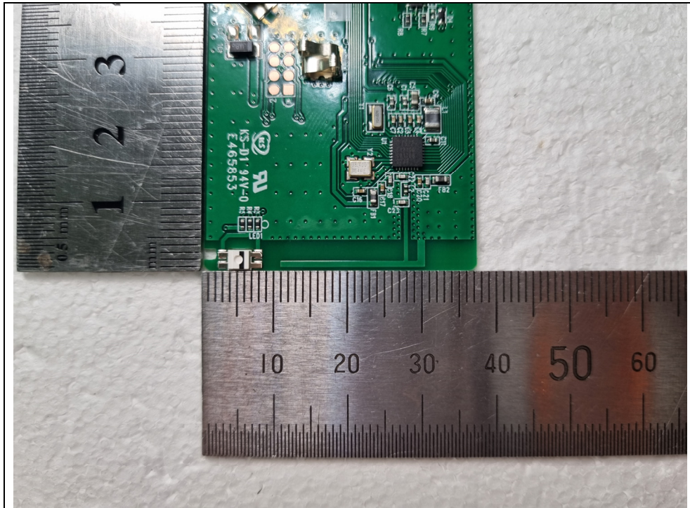
Antenna
