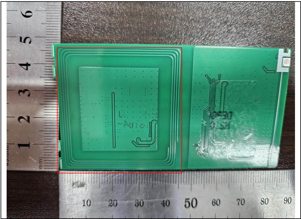
NFC Antenna
