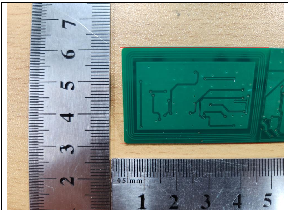
NFC Antenna
