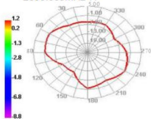
2500.000MHz H
