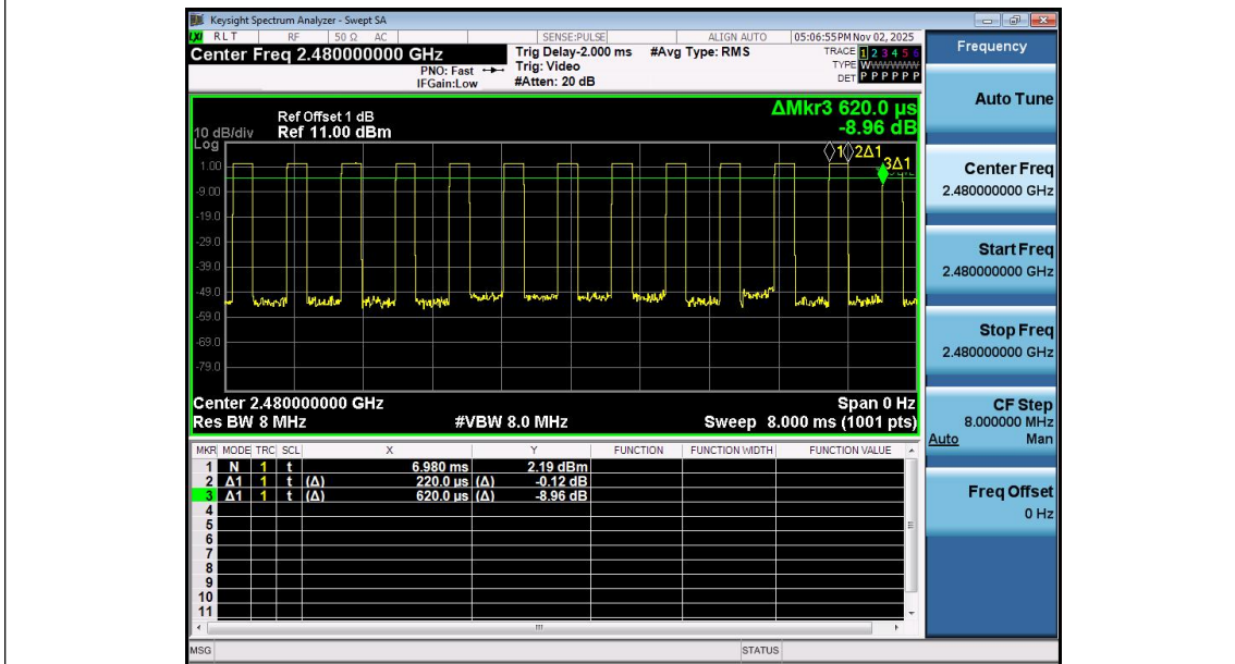
NTNV-BLE_2M-Ant1-2480
