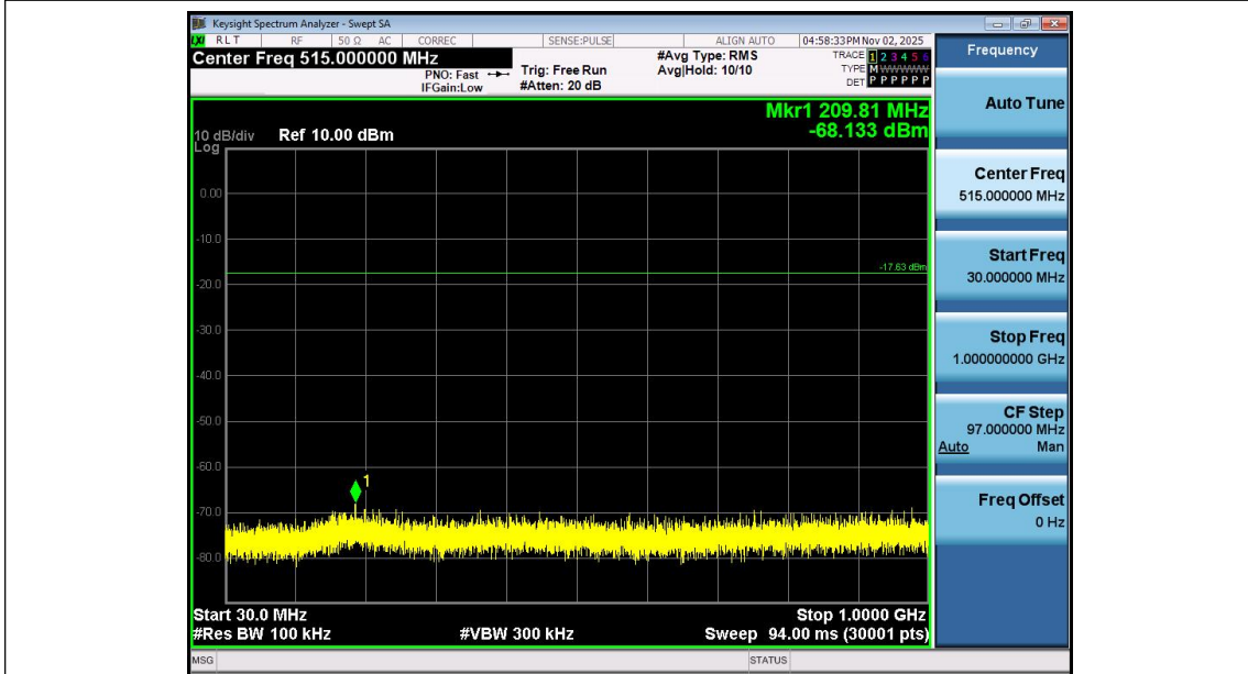
BLE_2M-Ant1-2440-30~1000-PASS
