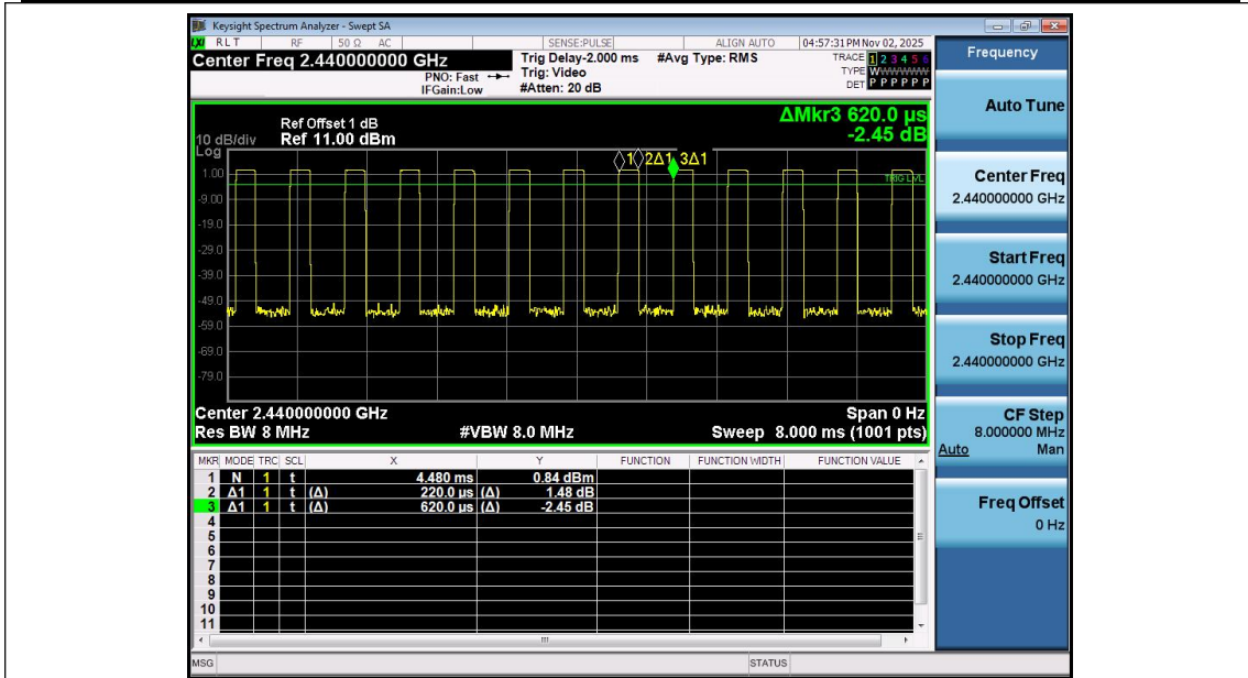
NTNV-BLE_2M-Ant1-2440
