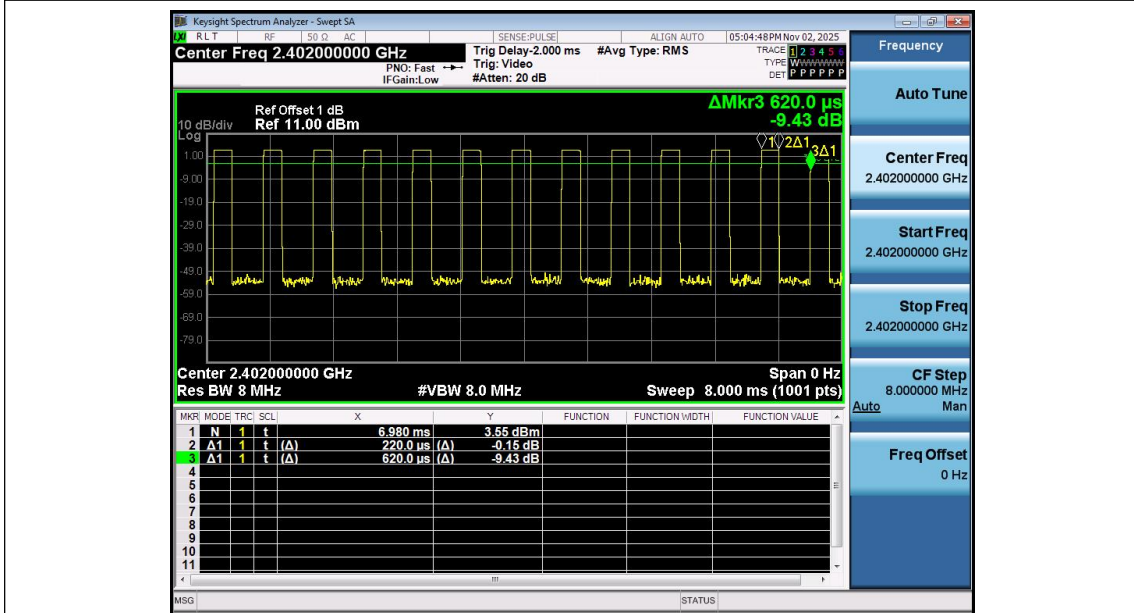
NTNV-BLE_2M-Ant1-2402
