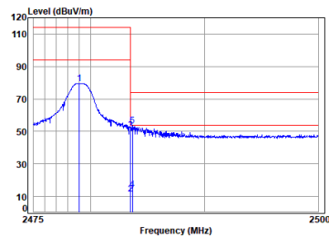
2.4G SRD_TX_CH_H_Vertical
