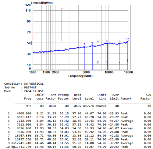
2.4G SRD_TX_CH_L_Vertical
