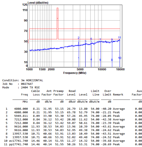
2.4G SRD_TX_CH_L_Horizontal
