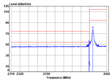
2.4G SRD_TX_CH_L_Vertical
