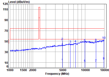
2.4G SRD_TX_CH_H_Horizontal
