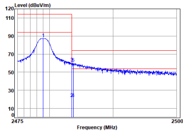
2.4G SRD_TX_CH_H_Horizontal
