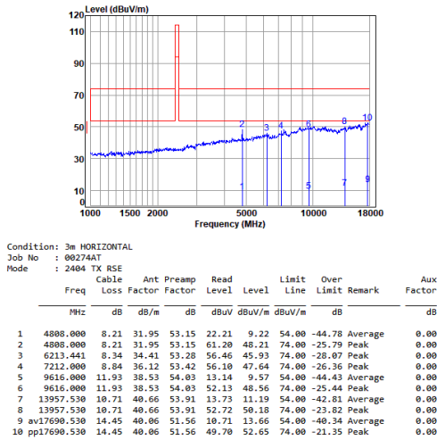
2.4G SRD_TX_CH_L_Horizontal
