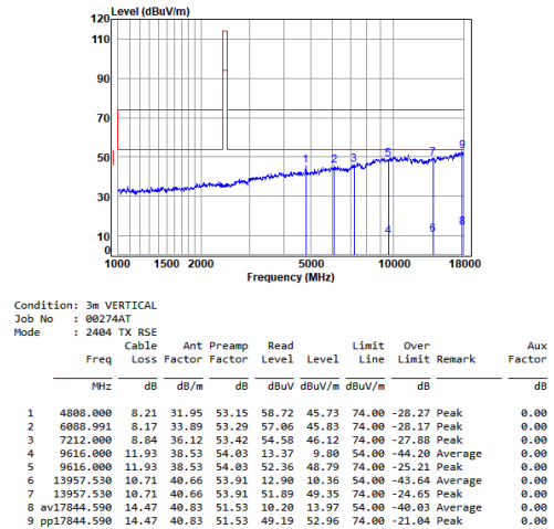
2.4G SRD_TX_CH_L_Vertical
