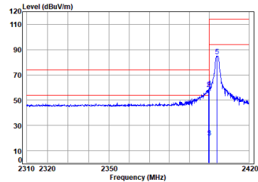
2.4G SRD_TX_CH_L_Vertical
