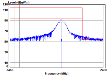
2.4G SRD_TX_CH_H_Horizontal
