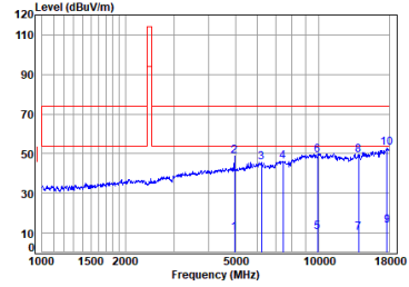
2.4G SRD_TX_CH_H_Vertical
