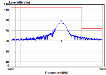
2.4G SRD_TX_CH_H_Vertical
