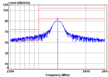
2.4G SRD_TX_CH_L_Horizontal
