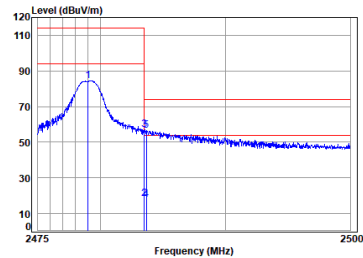
2.4G SRD_TX_CH_H_Vertical
