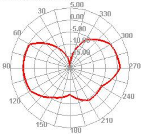
2450.000MHz E1
