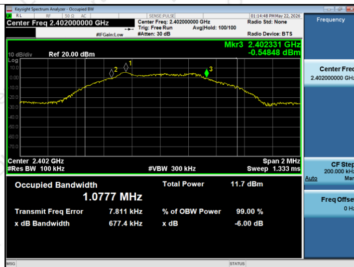
-6dB Bandwidth NVNT BLE 1M 2402MHz Ant1
