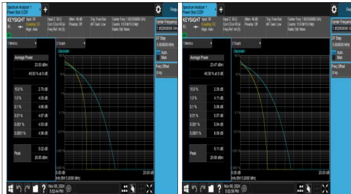
Band2-5MHz-16QAM-18625-1RB#0-PASS
