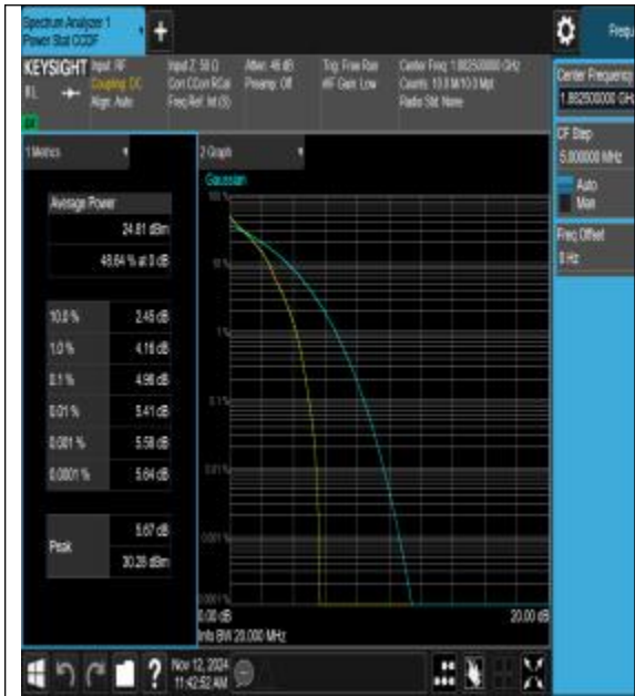
Band25-20MHz-QPSK-26365-1RB#0-PASS
