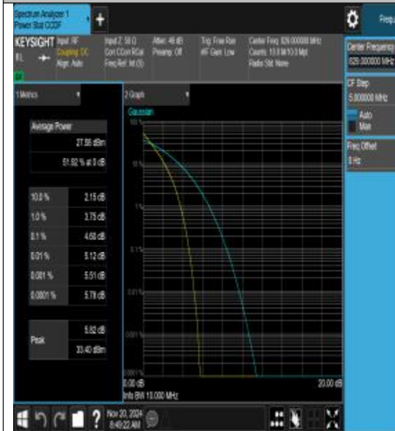
26(824-849)-10MHz-QPSK-26840-50RB#0-PASS
