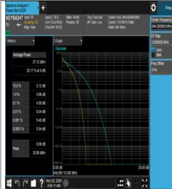
26(824-849)-10MHz-QPSK-26990-50RB#0-PASS
