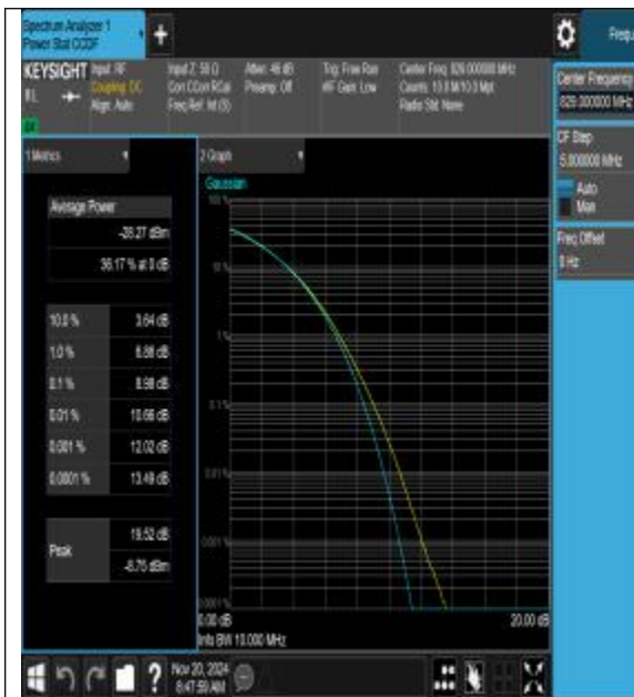
26(824-849)-10MHz-QPSK-26840-1RB#0-PASS
