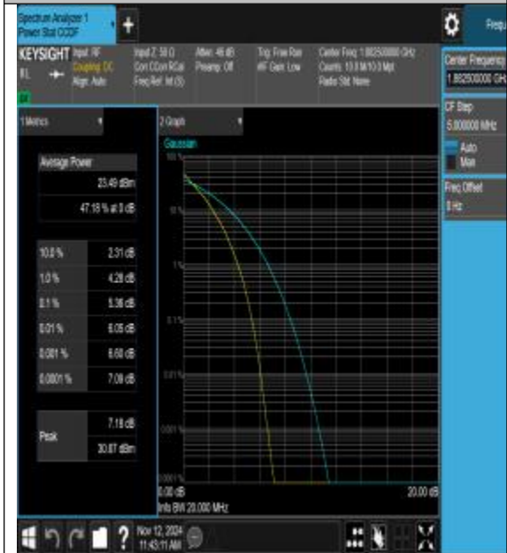
Band25-20MHz-QPSK-26365-100RB#0-PASS
