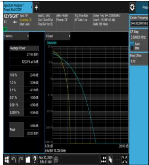
26(824-849)-10MHz-16QAM-26990-1RB#0-PASS
