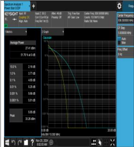
26(824-849)-10MHz-QPSK-26915-50RB#0-PASS
