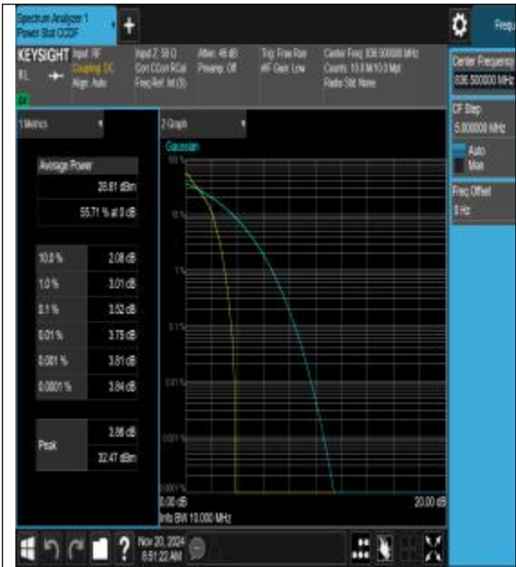
26(824-849)-10MHz-QPSK-26915-1RB#0-PASS
