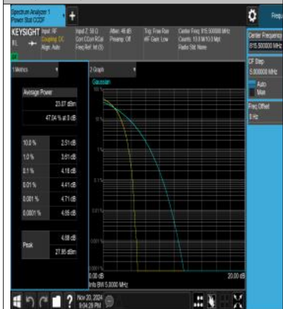
26(814-824)-3MHz-QPSK-26705-15RB#0-PASS
