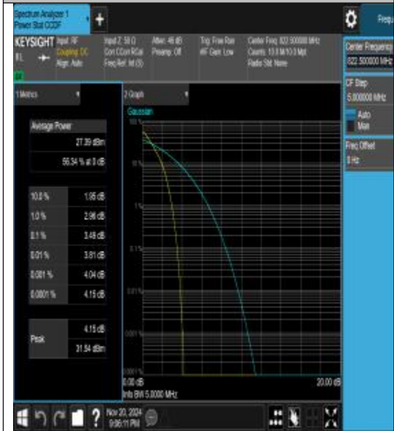
26(814-824)-3MHz-QPSK-26775-15RB#0-PASS
