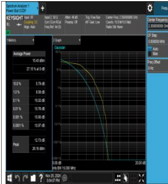
40(2345-2360)-10MHz-QPSK-39150-1RB#0-PAS
