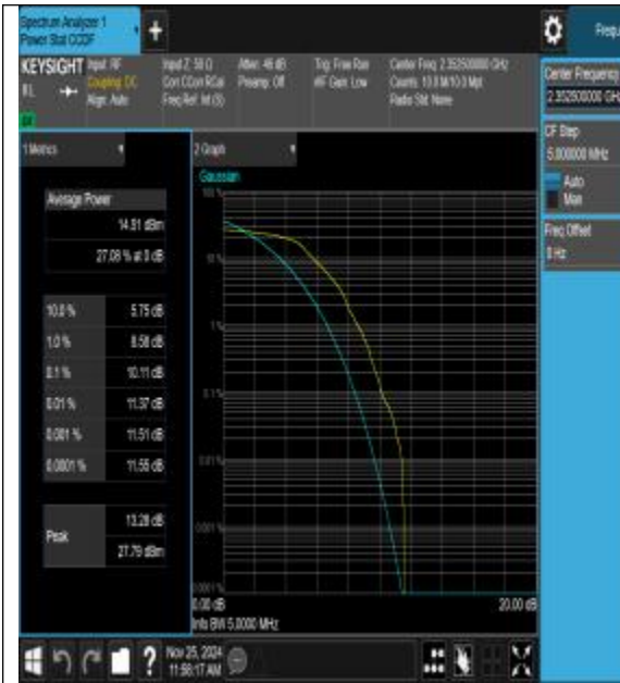
40(2345-2360)-5MHz-QPSK-39175-1RB#0-PASS
