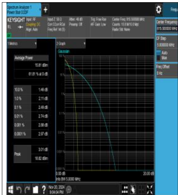
26(814-824)-3MHz-QPSK-26705-1RB#0-PASS
