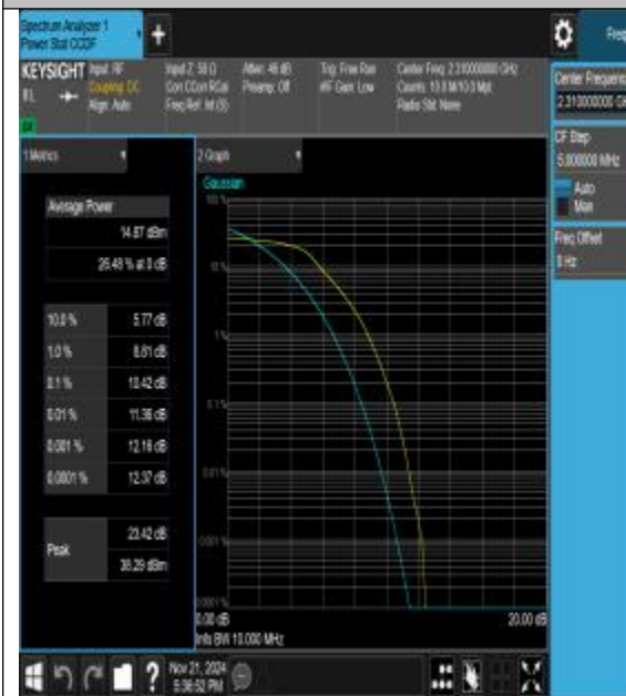
40(2305-2320)-10MHz-QPSK-38750-50RB#0-PA
