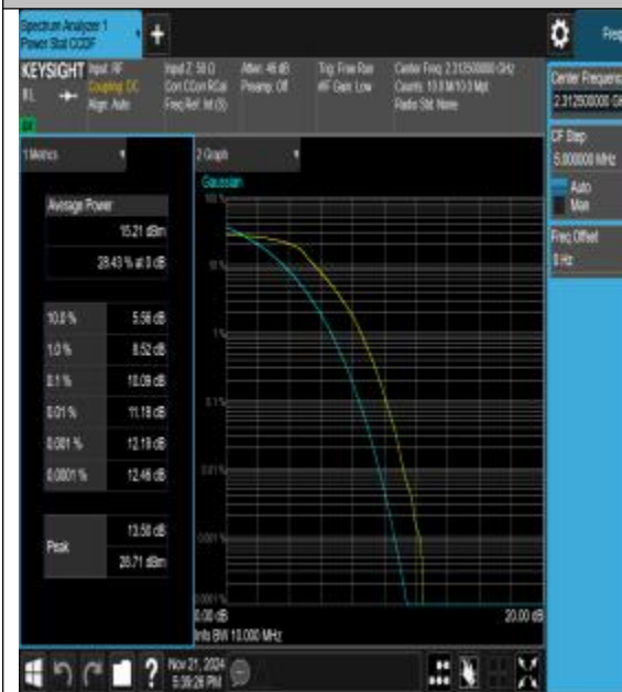
40(2305-2320)-10MHz-QPSK-38775-50RB#0-PA
