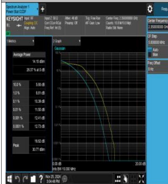
40(2345-2360)-10MHz-QPSK-39150-50RB#0-PA
