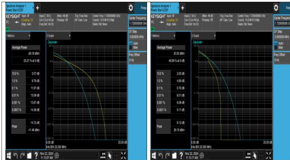
Band66-20MHz-QPSK-132072-1RB#0-PASS
