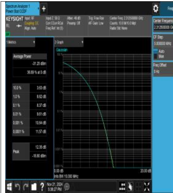
40(2305-2320)-10MHz-QPSK-38775-1RB#0-PAS
