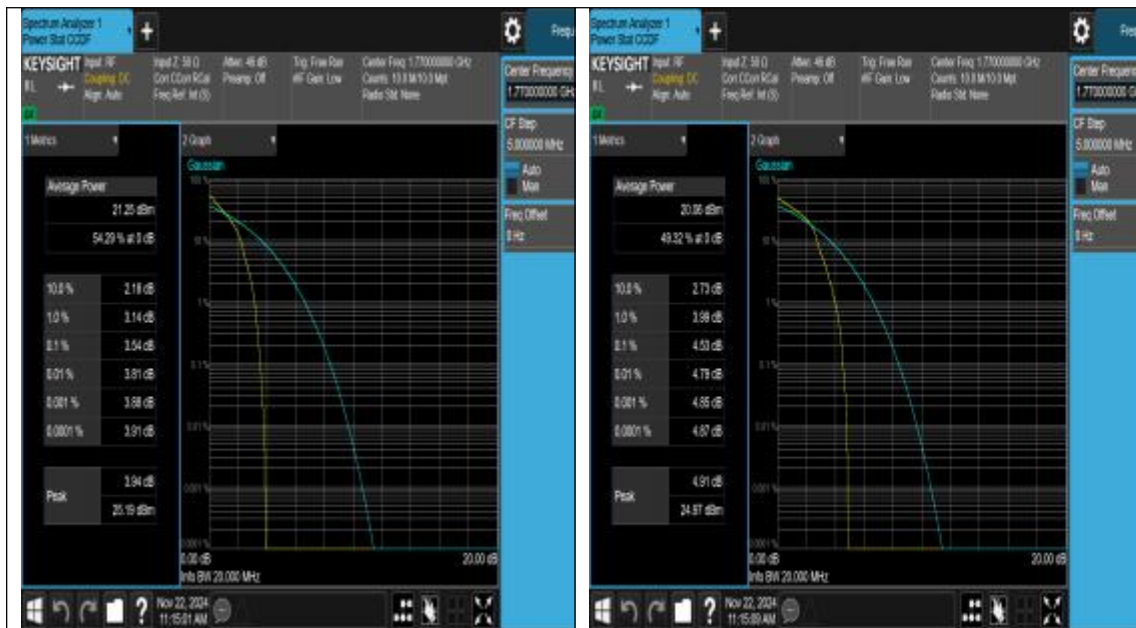
Band66-20MHz-QPSK-132572-1RB#0-PASS
