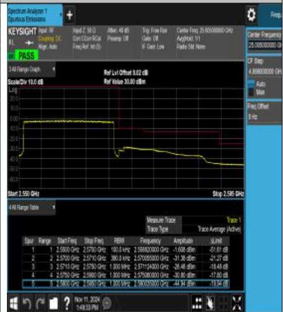
Band7_20MHz_16QAM_21350_100RB#0
