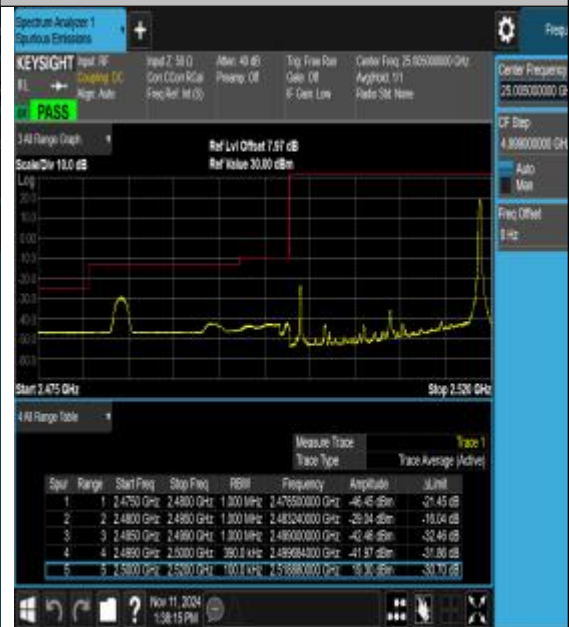
Band7_20MHz_16QAM_20850_1RB#99
