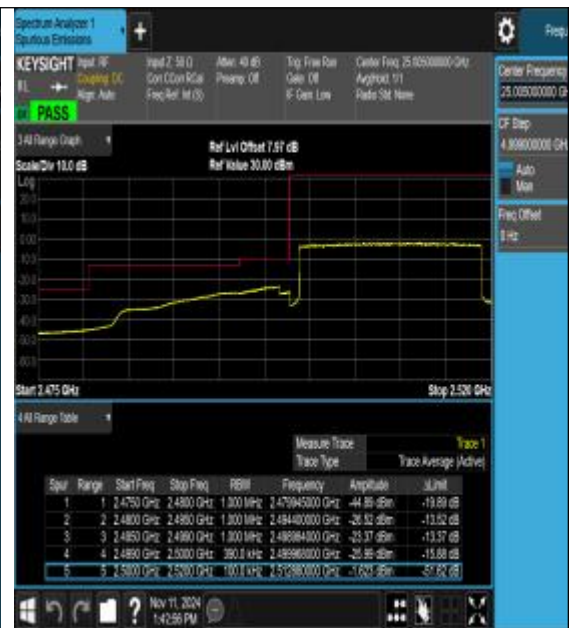
Band7_20MHz_16QAM_20850_100RB#0
