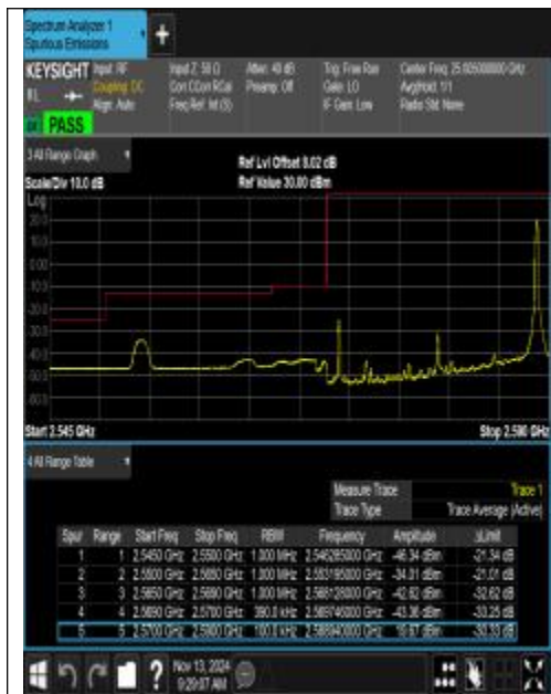
Band38_20MHz_QPSK_37850_1RB#99
