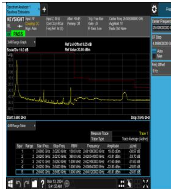
Band38_20MHz_QPSK_38150_1RB#0
