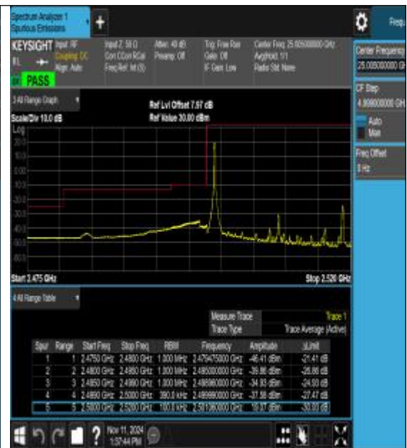
Band7_20MHz_16QAM_20850_1RB#0
