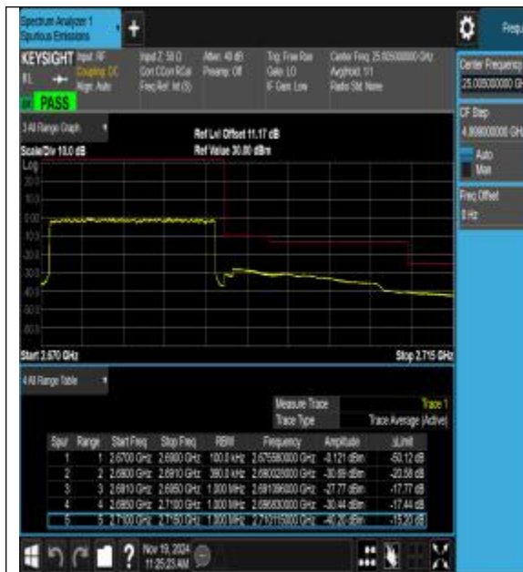
Band41_20MHz_QPSK_41490_100RB#0
