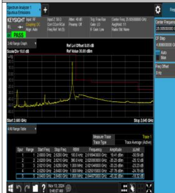
Band38_20MHz_QPSK_38150_1RB#99
