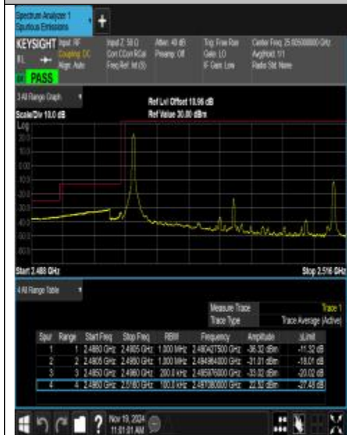
Band41_20MHz_QPSK_39750_1RB#0
