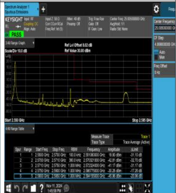
Band7_20MHz_16QAM_21350_1RB#0
