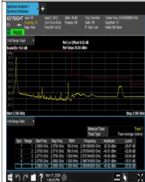
Band7_20MHz_QPSK_21350_1RB#0
