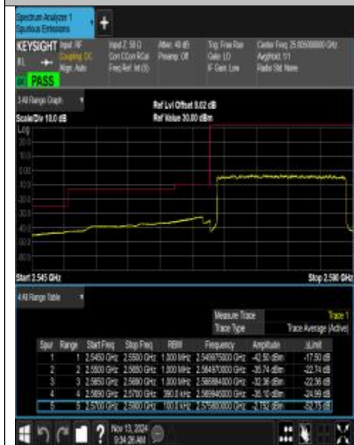
Band38_20MHz_QPSK_37850_100RB#0
